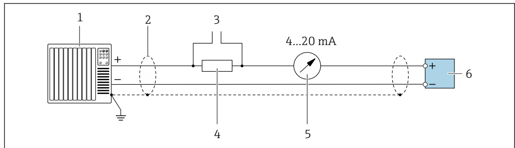
图 17 4...20 mA HART 电流输出 (有源) 的接线图
