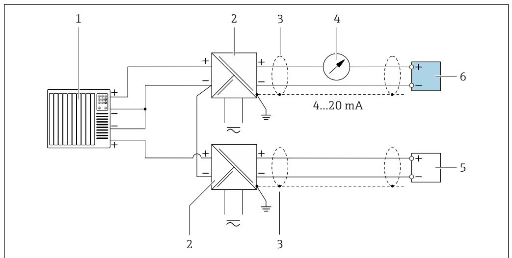
图 19 接线实例：HART 输入，公共端接负极（无源信号）
