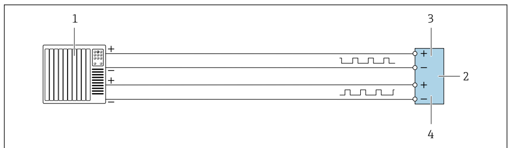
22 Exemple de raccordement pour la double sortie impulsion (active)
