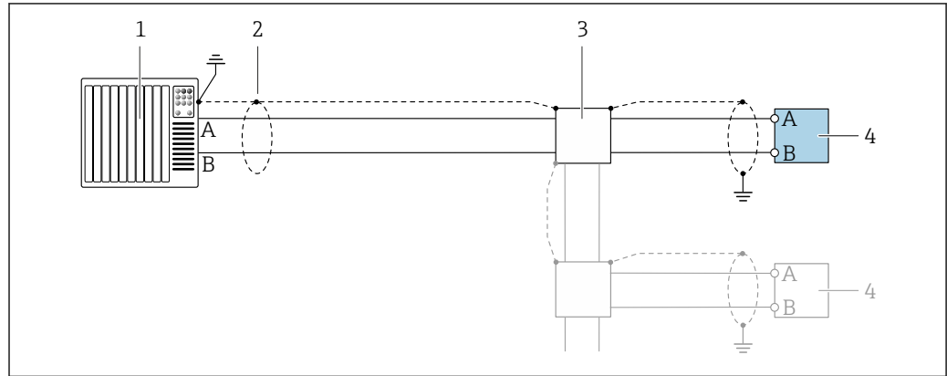
17 Exemple de raccordement pour Modbus RS485, zone non explosible et Zone 2 ; Class I, Division 2
