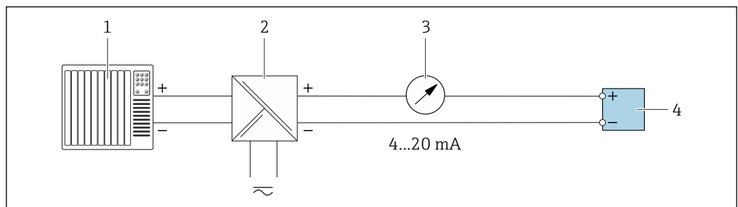
图 19 接线实例：4...20 mA 电流输出（无源信号）
