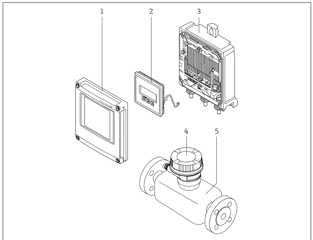
☑ 1 仪表的主要组成部件
