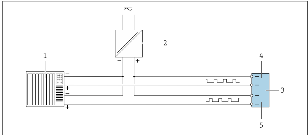
图 23 接线实例：双脉冲输出（无源信号）
