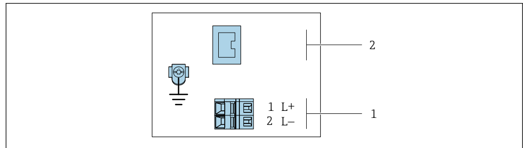
图 7 EtherNet/IP 型设备的接线端子分配示意图
