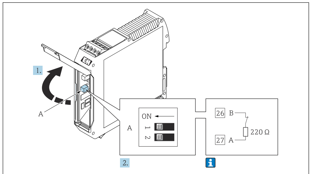
17 La résistance de fin de ligne peut être activée via le commutateur DIP dans la barrière de sécurité Promass 100
