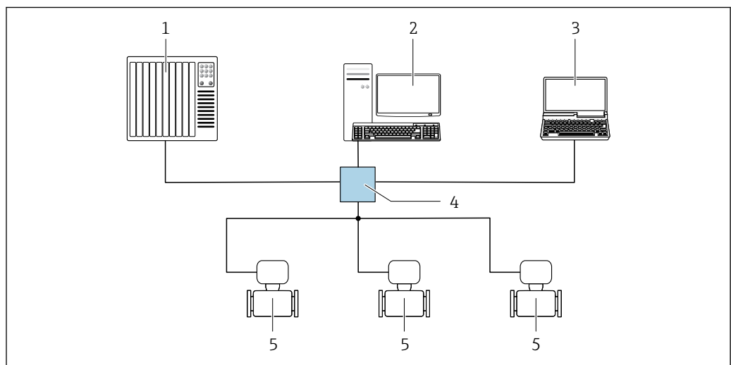
13 Options pour la configuration à distance via le réseau EtherNet/IP : topologie en étoile
