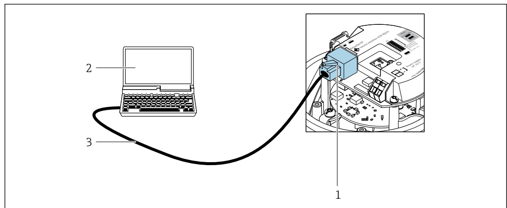
■ 18 Raccordement pour caractéristique de commande "Sortie", option N : EtherNet/IP
