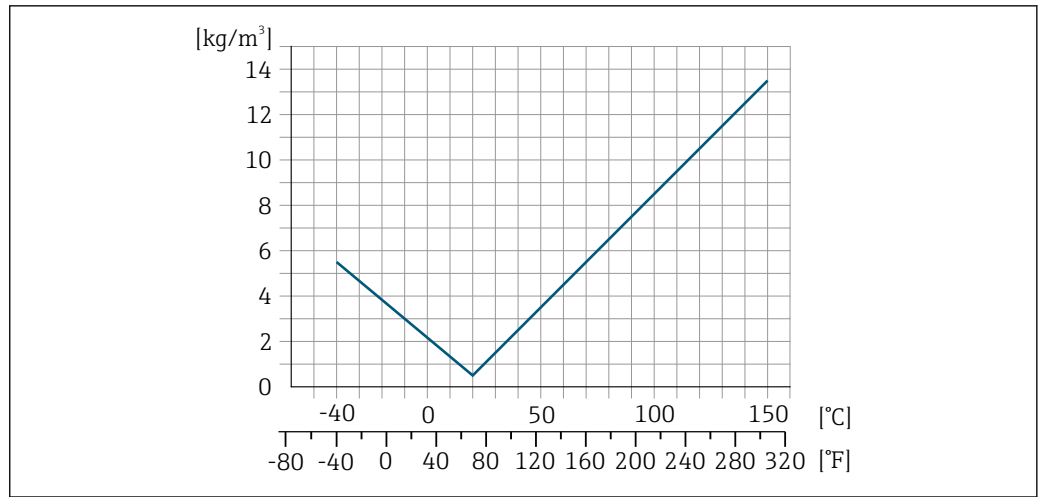
15 Ajustage sur site de la masse volumique, par exemple à +20 °C (+68 °F)
