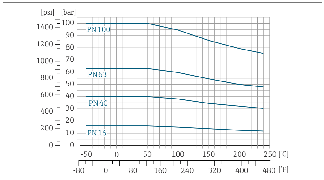
15 Avec matériau de bride 1.4404 (F316/F316L), Alloy C22
