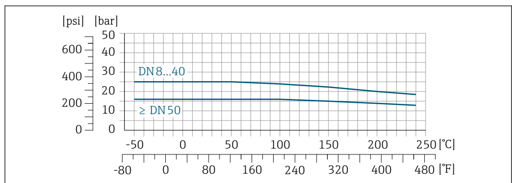
19 Avec matériau de raccord 1.4404 (316/316L)
