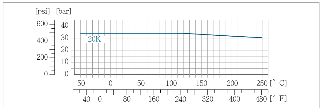
22 Avec matériau de bride 1.4301 (F304) ; pièces en contact avec le produit Alloy C22
