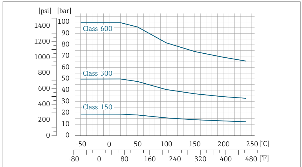
21 Avec matériau de bride 1.4301 (F304) ; pièces en contact avec le produit Alloy C22
