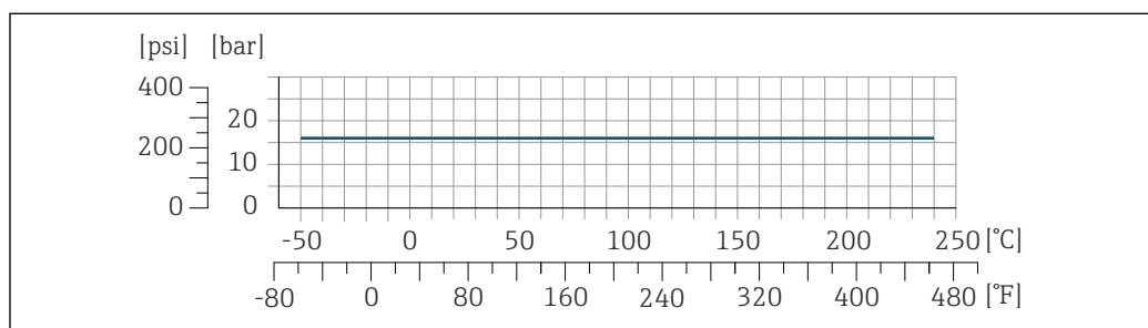
25 Avec matériau de raccord 1.4404 (316/316L)
