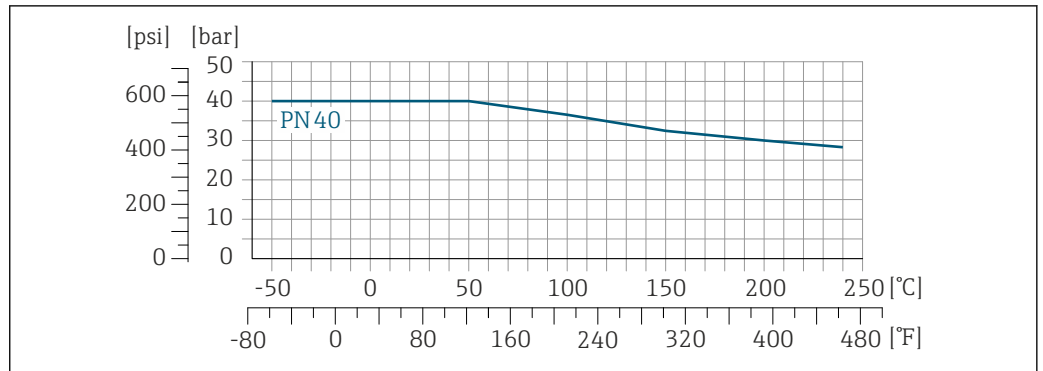
20 Avec matériau de bride 1.4301 (F304) ; pièces en contact avec le produit Alloy C22
