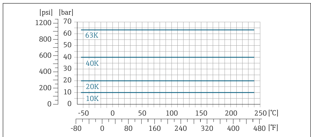
18 Avec matériau de bride 1.4404 (F316/F316L), Alloy C22
