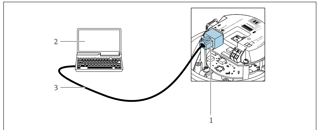
14 Connexion pour la caractéristique de commande "Sortie", option R : PROFINET
