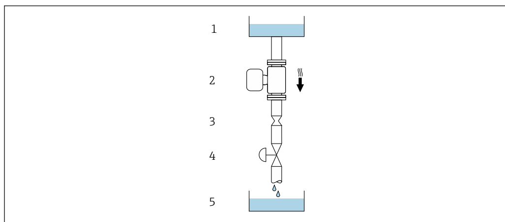
5 Montage dans un écoulement gravitaire (p. ex. applications de dosage)
