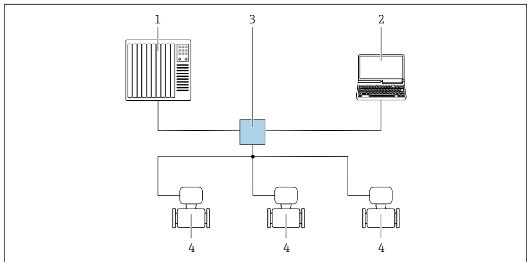
📄 13 Options de configuration à distance via réseau PROFINET : topologie en étoile
