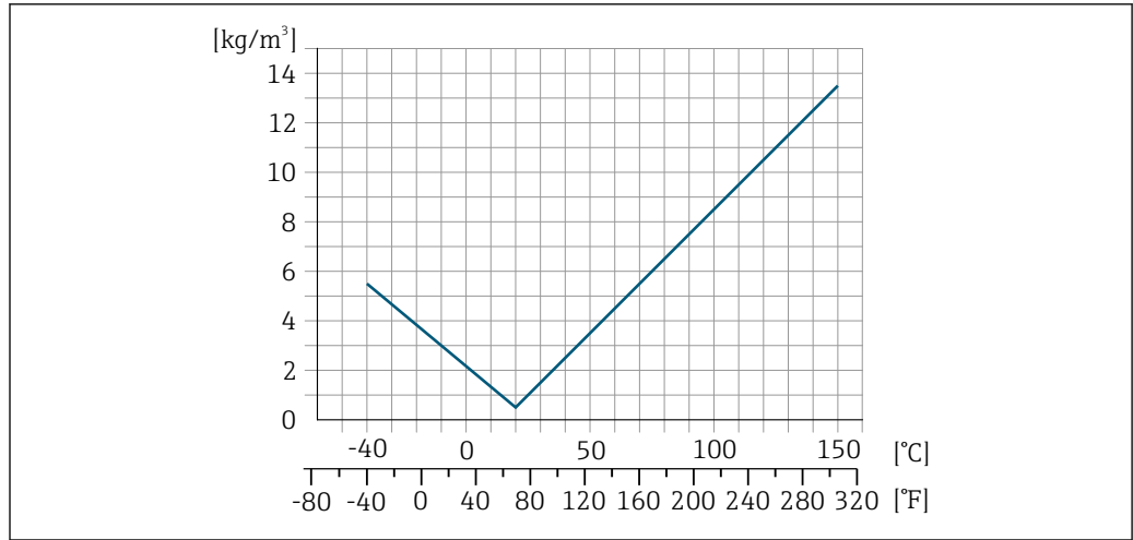
16 Ajustage sur site de la masse volumique, par exemple à +20 °C (+68 °F)
