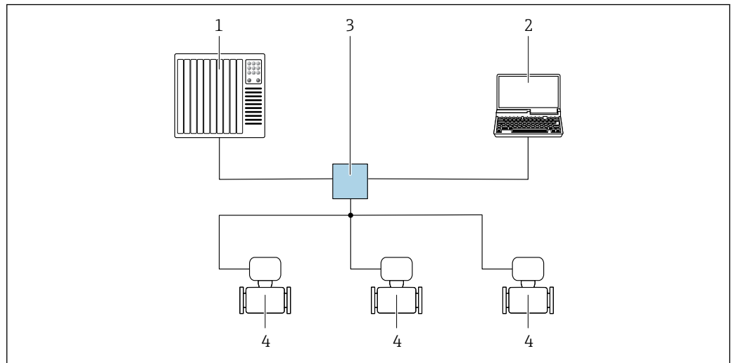
18 Options de configuration à distance via réseau PROFINET : topologie en étoile
