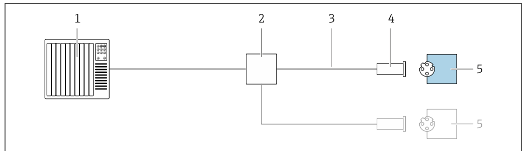
11 Exemple de raccordement pour PROFINET
