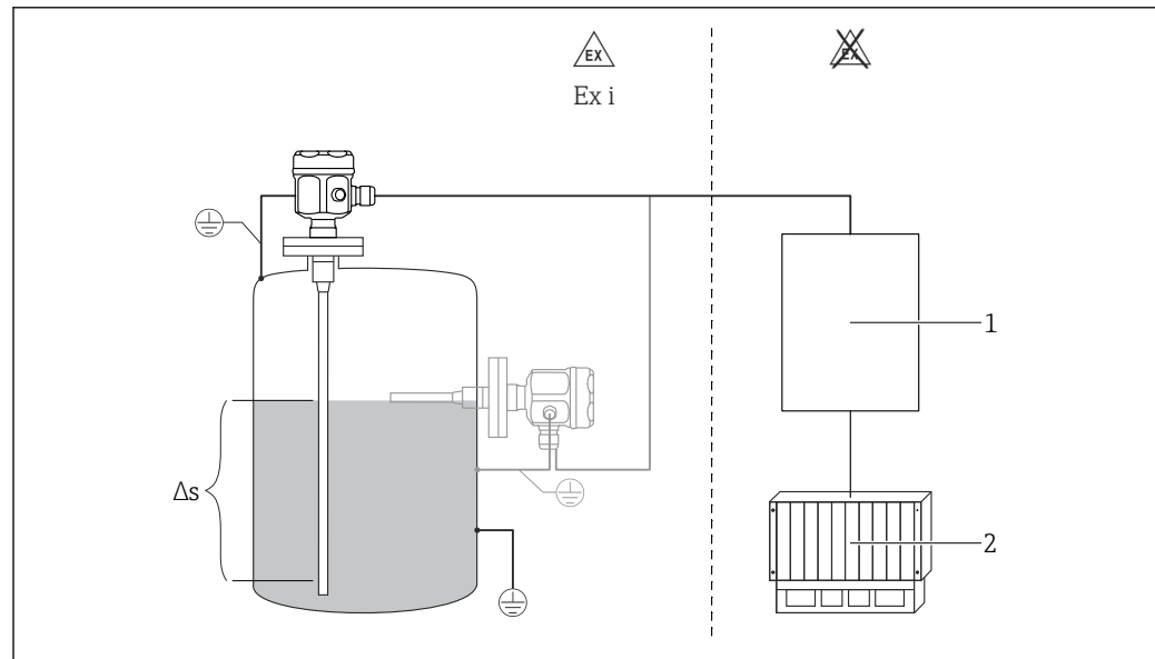
7 Sonde als Füllstandsgrenzschalter 8 ... 16 mA
