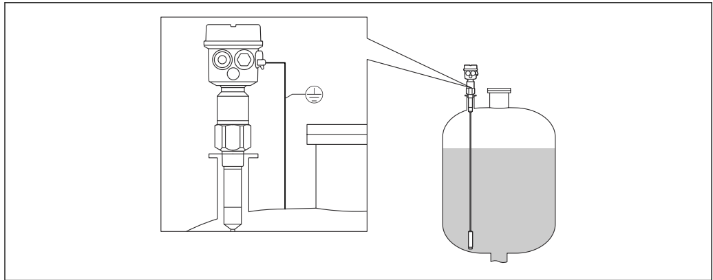
5 Uma sonda com comprimento de isolamento completamente inativo para bocais de instalação
