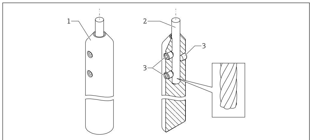
14 Aperçu du contrepois tenseur
