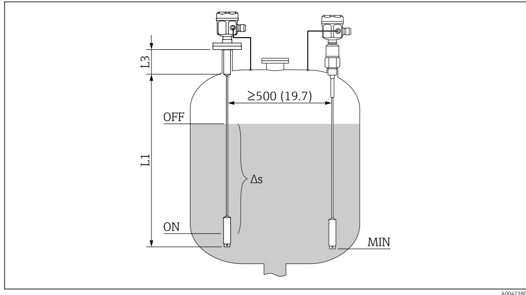
7 Condition de mesure. Unité de mesure mm (in)
