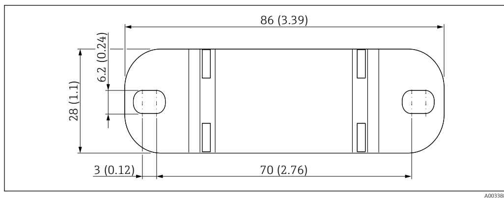
15 Visión general de la placa de montaje en pared. Unidad de medida mm (in)
