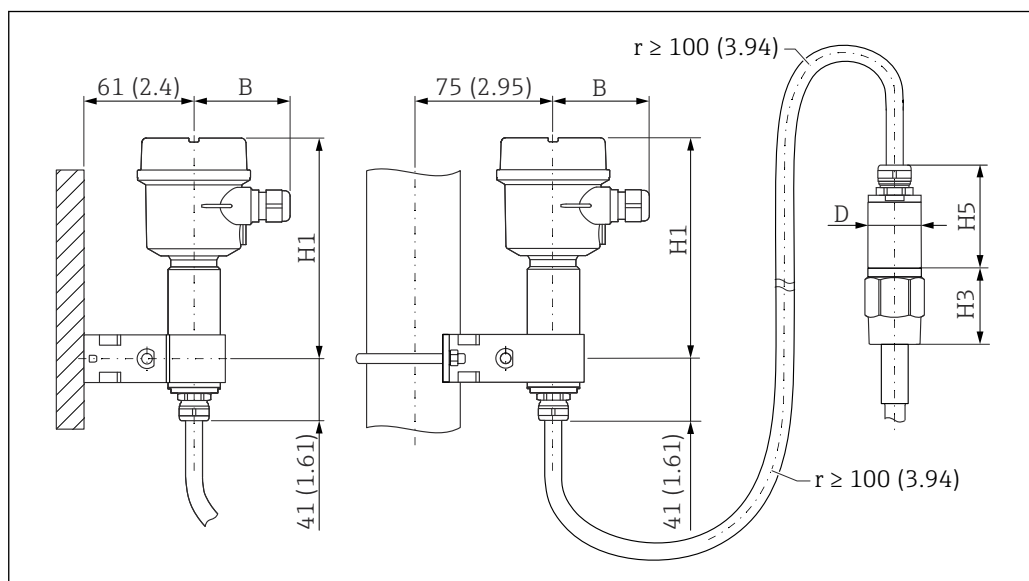
14 Côté boîtier : montage mural, montage sur conduite et côté capteur. Unité de mesure mm (in)
