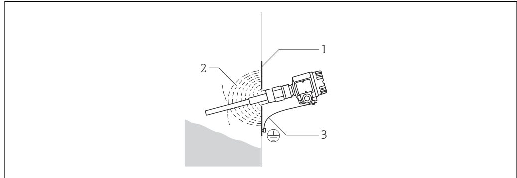
12 Sonde montée dans la paroi en plastique
