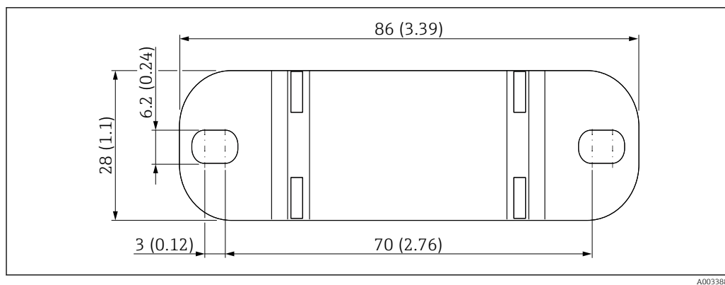
15 Aperçu de support mural. Unité de mesure mm (in)
