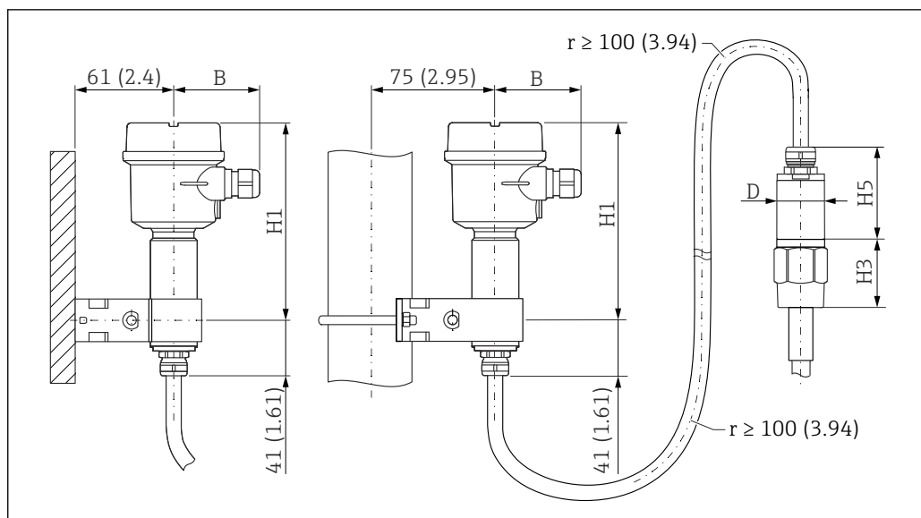
図 16 ハウジング側：壁面取付、パイプ取付、およびセンサ側。測定単位 mm (in)
