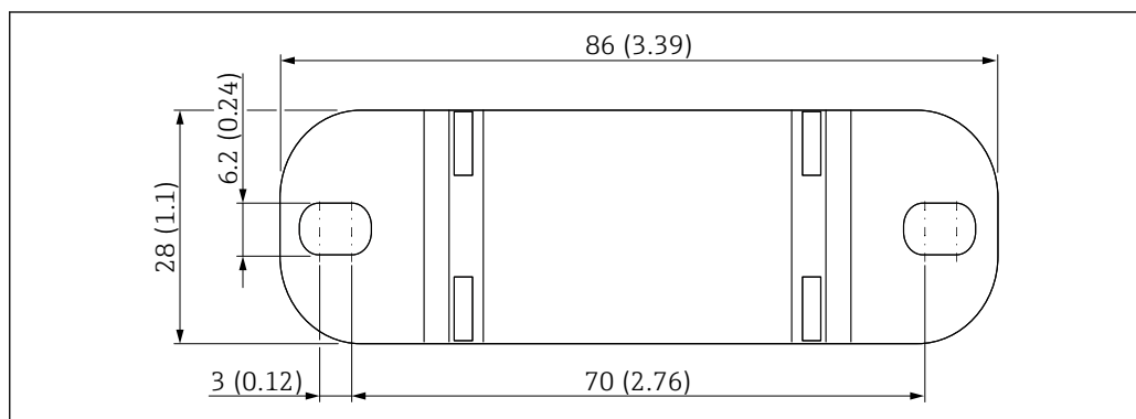
図 17 壁面取付ブラケットの概要。測定単位 mm (in)
