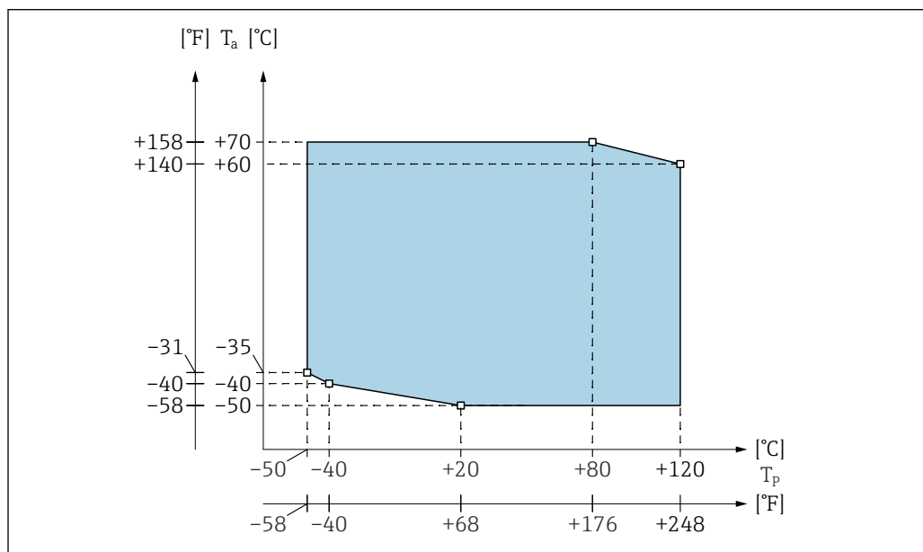
図 19 プロセス温度範囲図：完全絶縁プローブ
