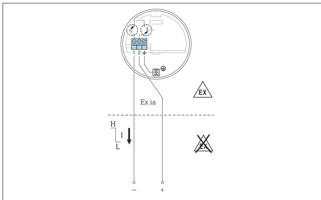
図 24 端子は、IEC 60947-5-6 (NAMUR) に準拠した変換器（絶縁アンプ）に接続してください
