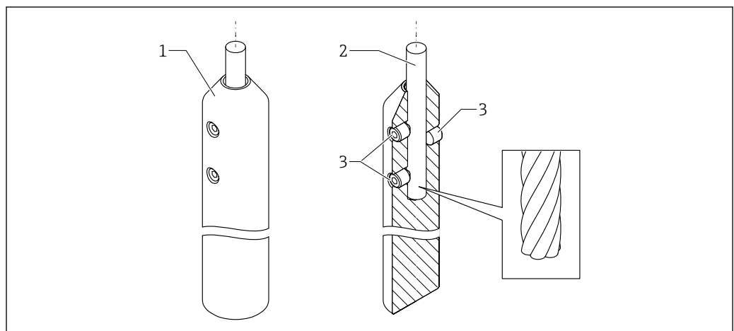
図 14 テンションウェイトの概要
