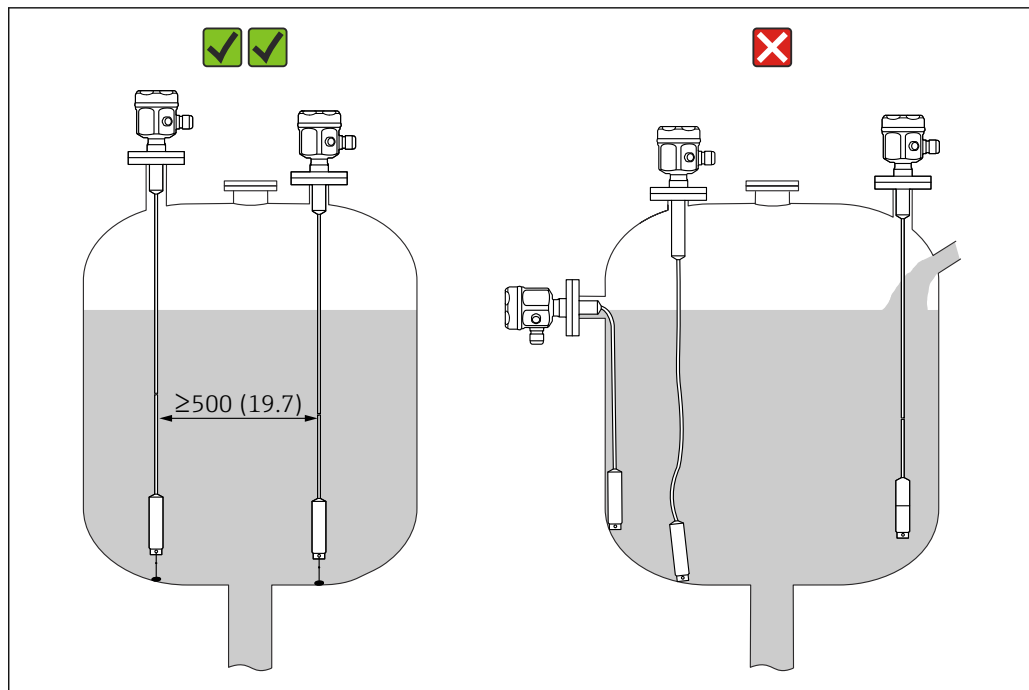
図 10 適切なプローブの取付け。測定単位 mm (in)
