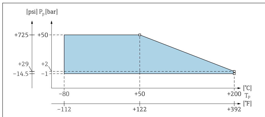
図 22 完全絶縁不感帯付きローブプローブの圧力および温度ディレーティング図
