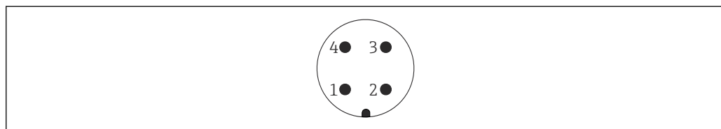
☒ 8 M12 コネクタ : 2 線式エレクトロニックインサート FEI55、FEI57、FEI58、FEI57C
