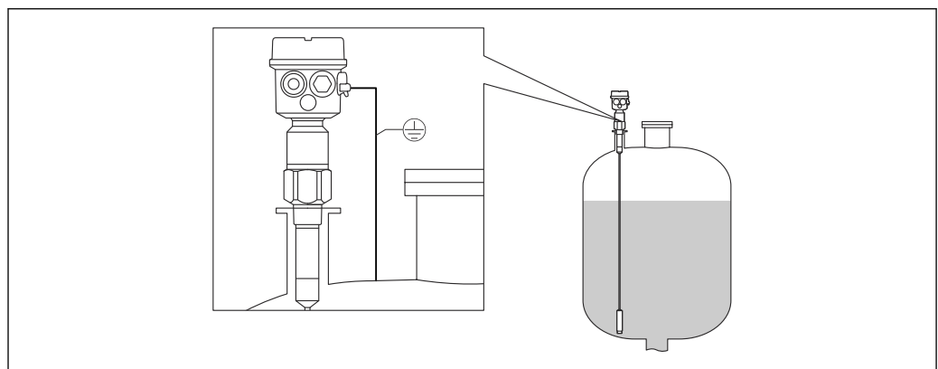
図 13 完全絶縁不感帯付きプローブ
