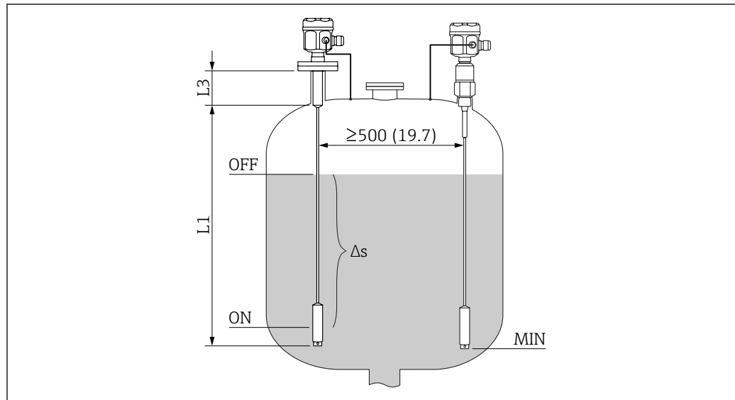
図 7 測定条件。測定単位 mm (in)
