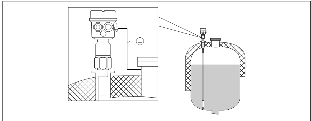
図 12 絶縁タンク用の不感帯付きプローブ
