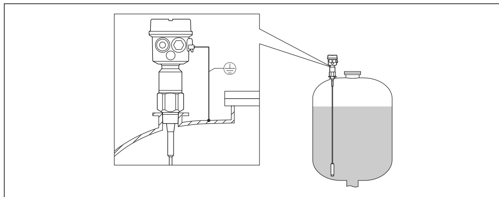
図 11 プローブおよび導電性タンク
