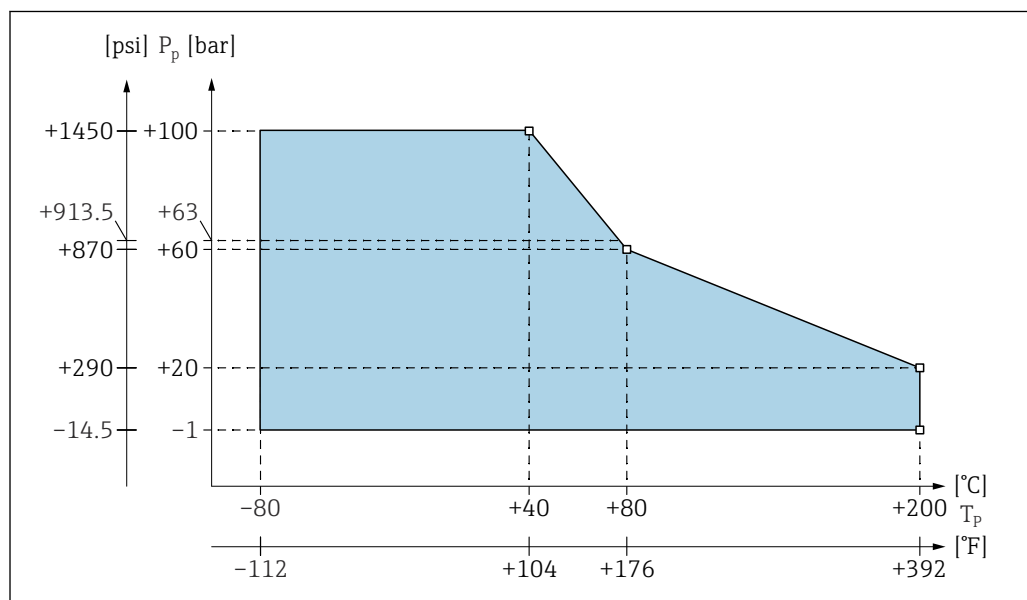
図 21 不感帯なし/不感帯付きローブプローブの圧力および温度ディレーティング図
