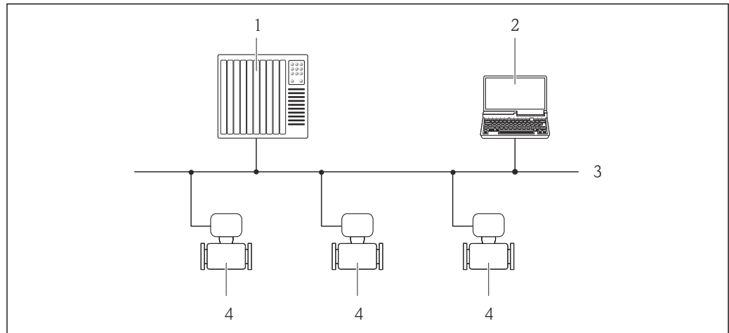
图 14 通过 PROFIBUS DP 网络进行远程操作
