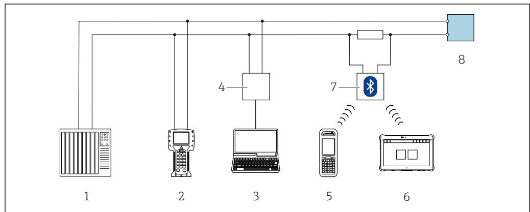
20 通过 HART 通信实现远程操作
