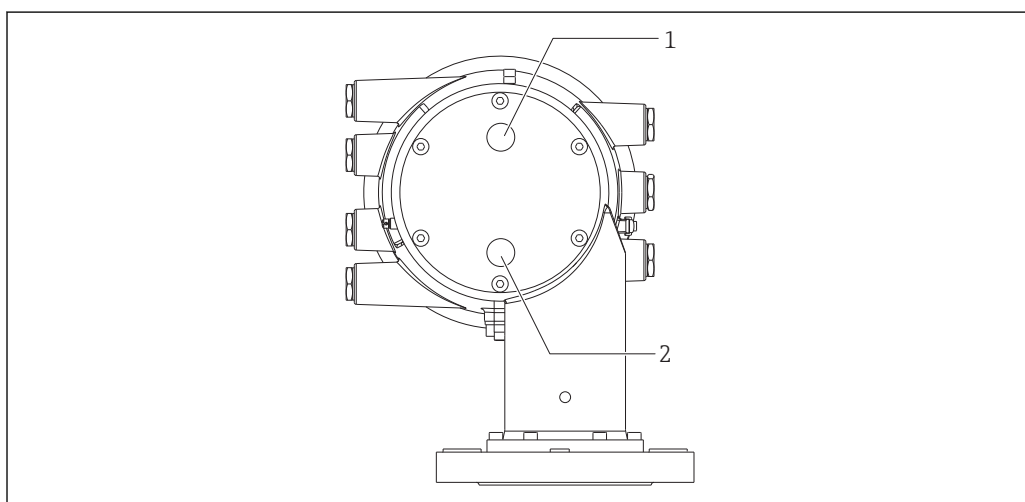
图 24 清洗短管和气体吹扫短管的连接孔口
