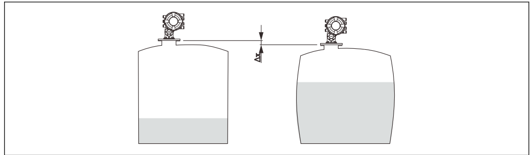
图 19 静压力导致罐体外壳膨胀，从而引起罐体参考高度位移 \Delta x
