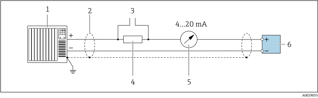
图 8 4...20 mA HART 电流输出(有源)的连接实例
