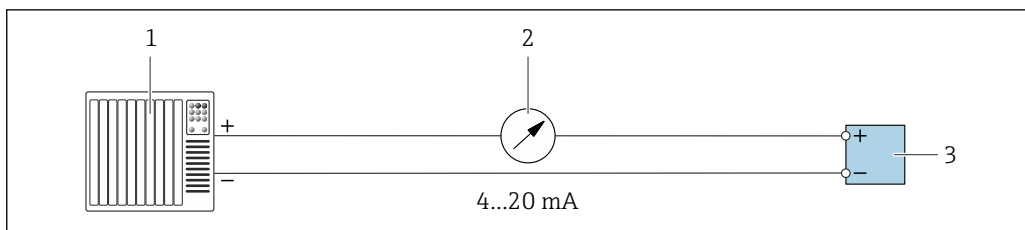
11 4...20 mA 有源电流输出的连接实例
