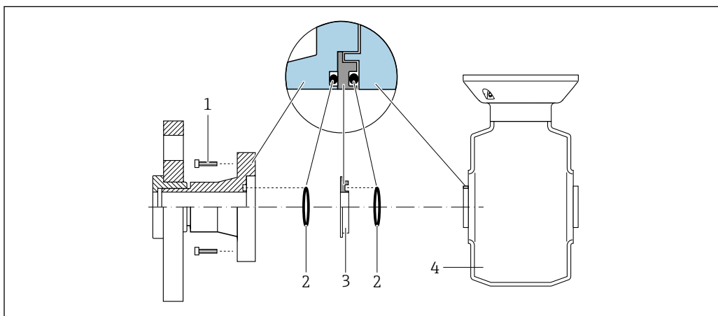
图 6 安装接地环
