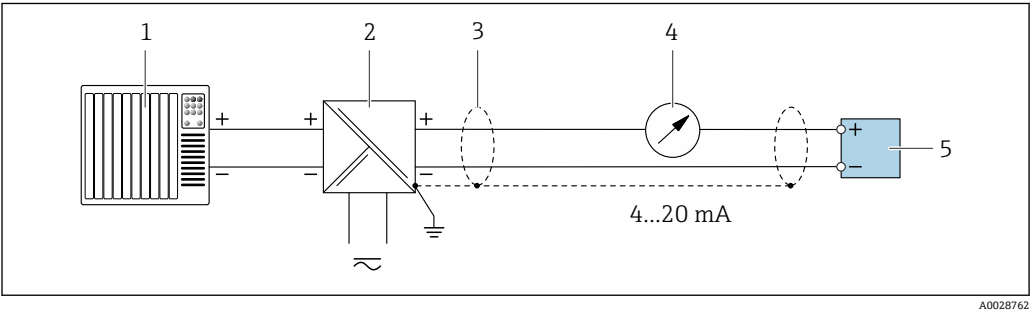
图 9 4...20 mA HART 电流输出(无源)的连接示例
