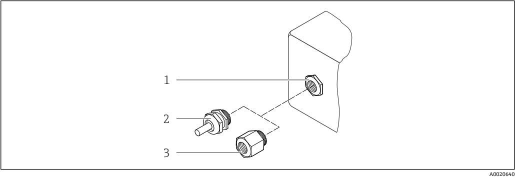
图 34 允许的电缆入口/缆塞 1 M20 × 1.5 内螺纹电缆入口 2 M20 × 1.5 缆塞 3 适配接头，适用于带 G ½"和 NPT ½"内螺纹的电缆入口
