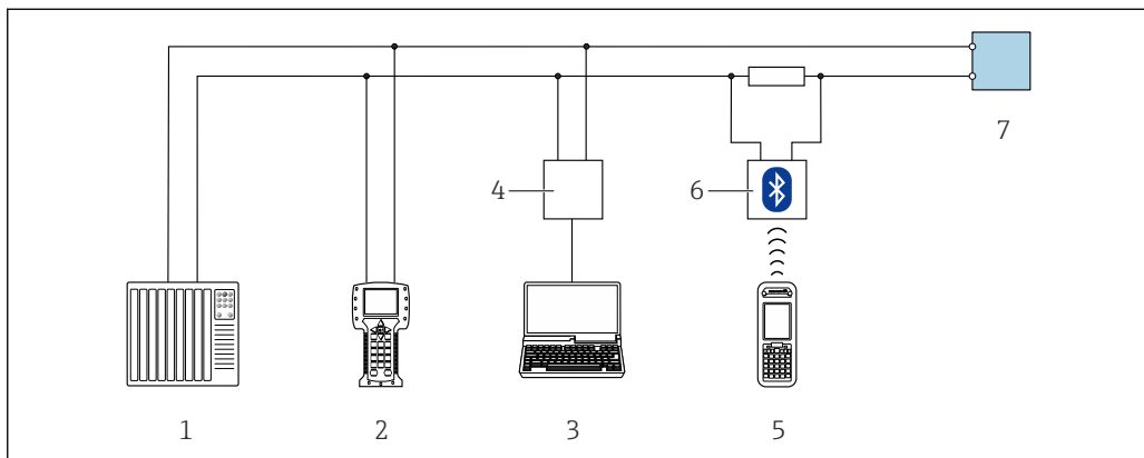
图 22 通过 HART 通信进行远程操作(有源信号)
