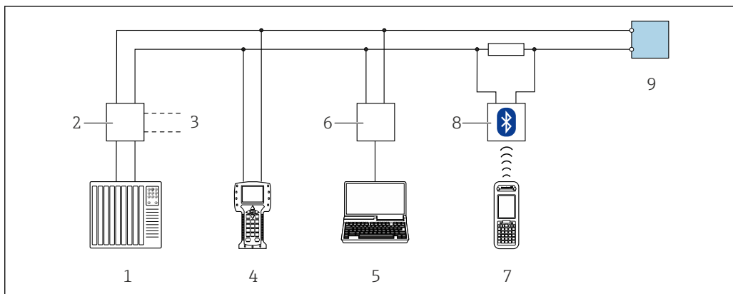
图 23 通过 HART 通信进行远程操作(无源信号)
