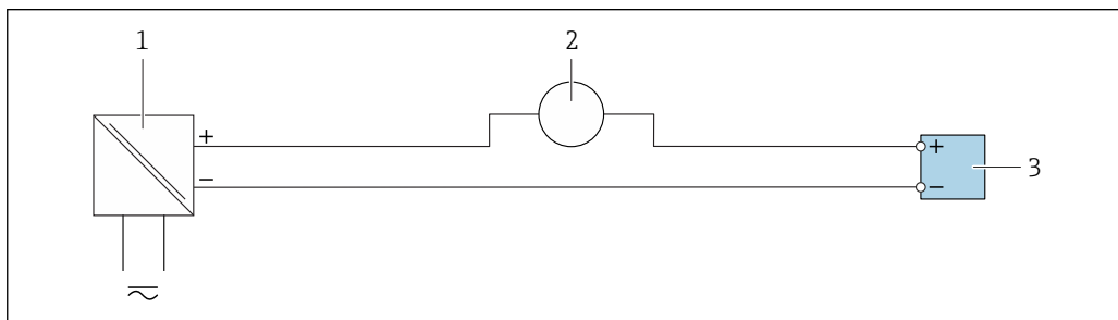
图 18 4...20 mA 电流输入的连接实例
