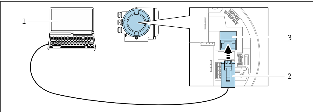
图 24 通过服务接口 (CDI-RJ45) 操作
