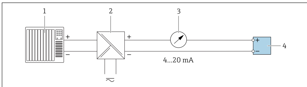
12 4...20 mA 无源电流输出的连接实例
