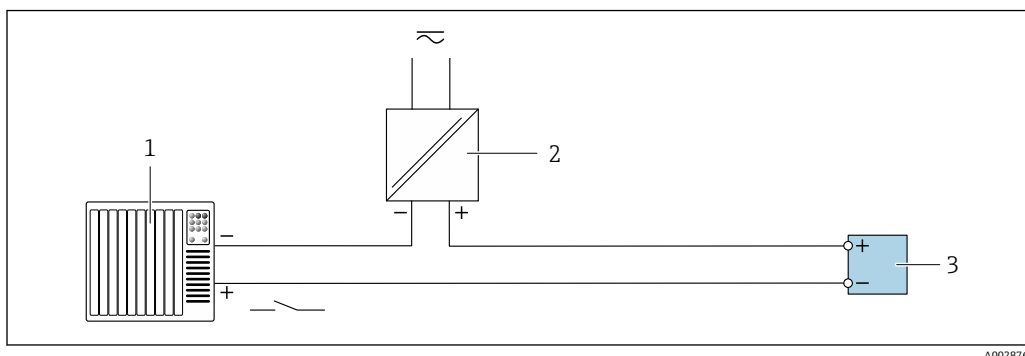
19 状态输入的连接实例
