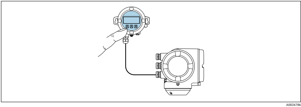
图 36 通过分离型显示与操作单元 DKX001 操作
