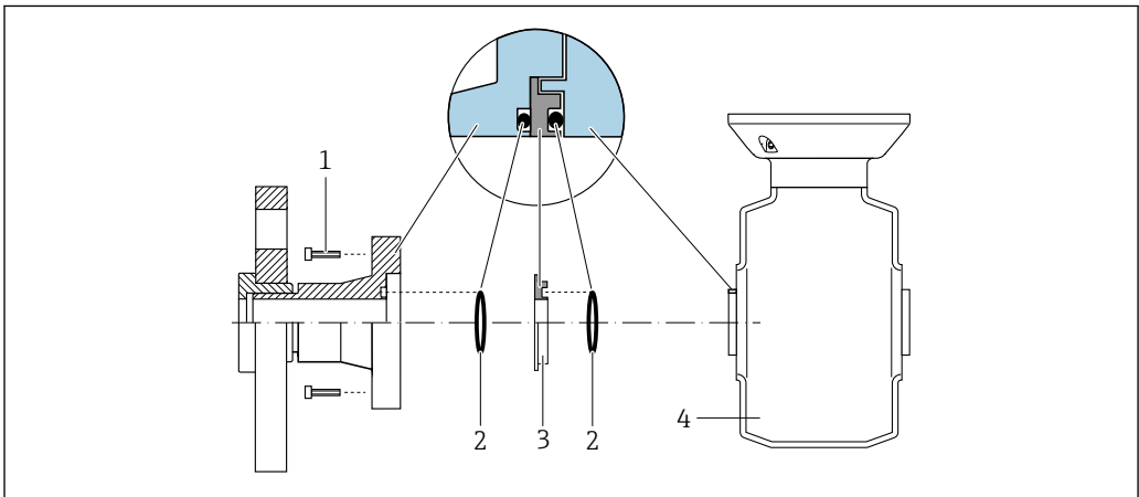
图 6 安装接地环
