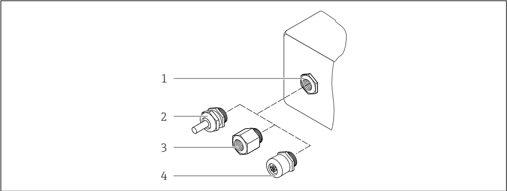
图 29 允许的电缆入口/缆塞 1 M20 × 1.5 内螺纹电缆入口 2 M20 × 1.5 缆塞 3 适配接头，适用于带 G ½"和 NPT ½"内螺纹的电缆入口 4 仪表插头
