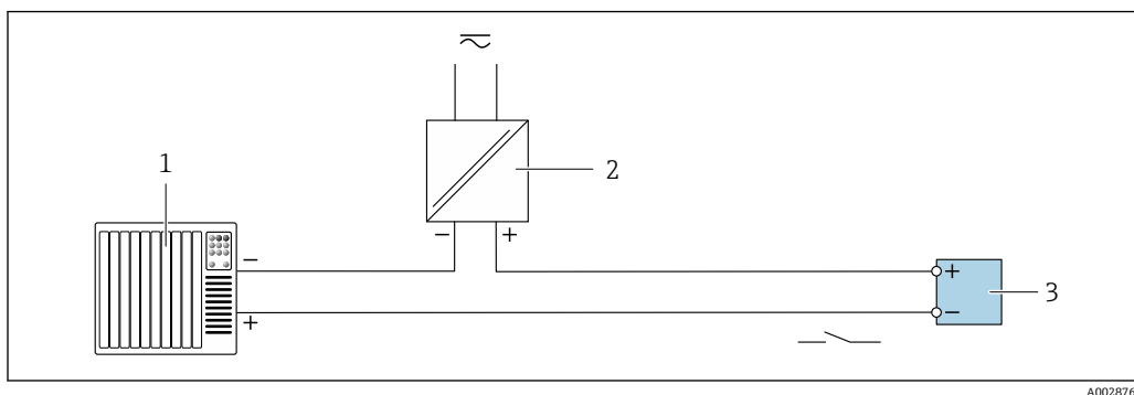
图 12 开关量输出(无源信号)的连接实例
