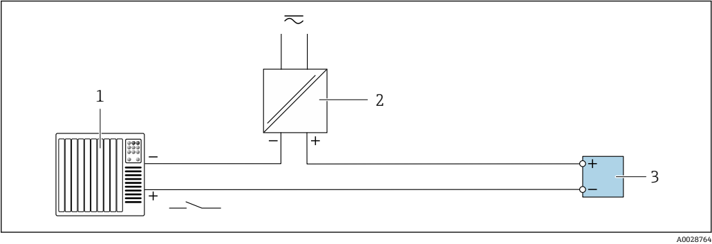
图 15 状态输入的连接实例
