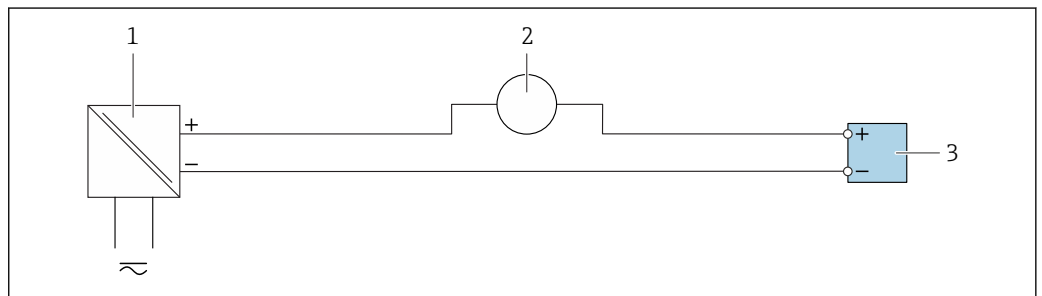
图 24 4...20 mA 电流输入的连接实例
