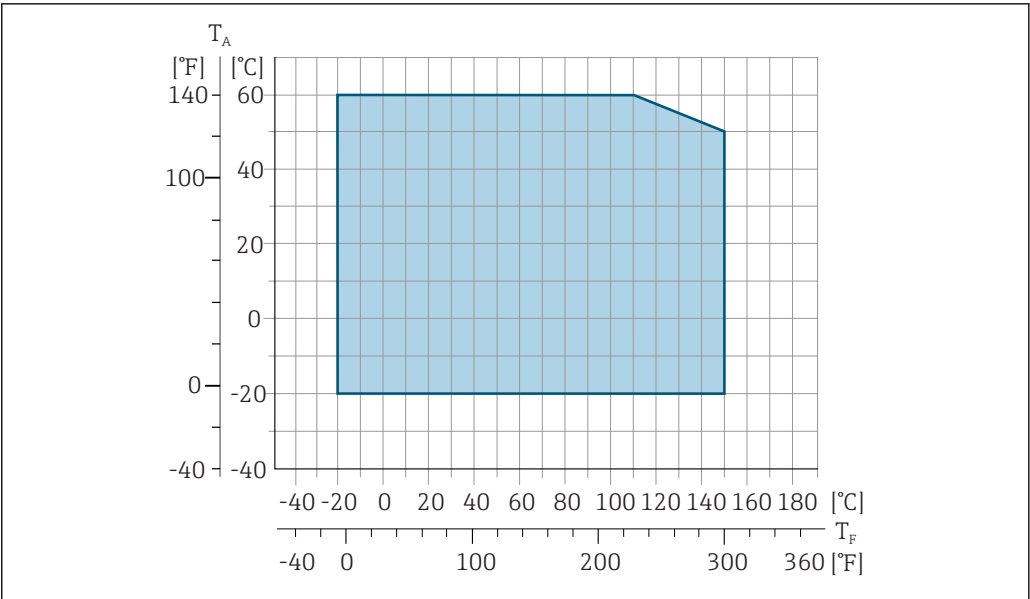
40 Promag 500 (数字式)
