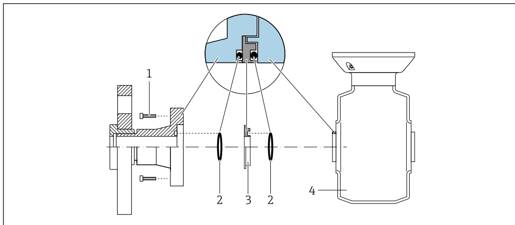
图 10 安装接地环
