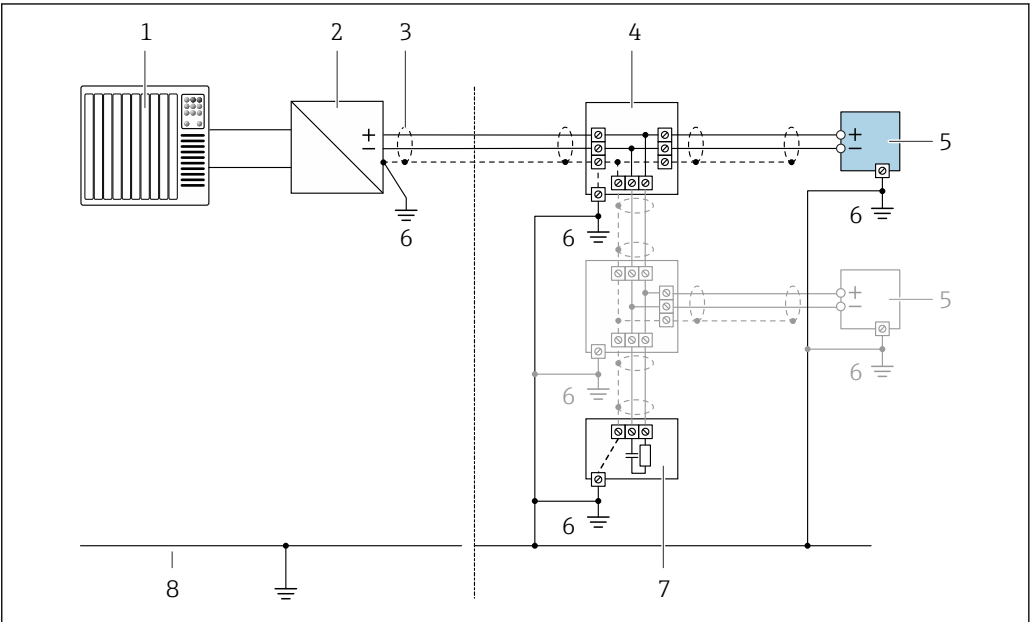
图 18 PROFIBUS PA 的连接实例
