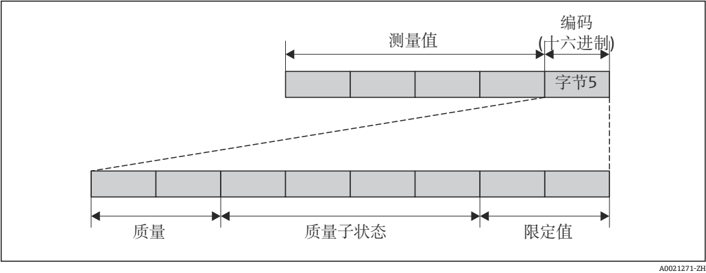
图 36 编码字节的结构
