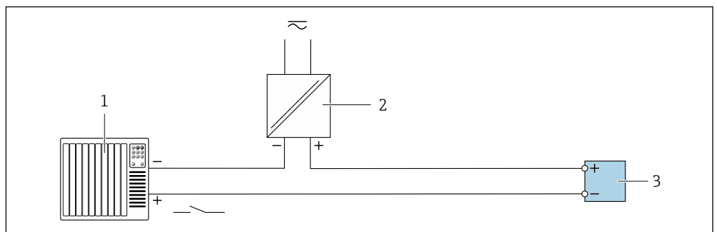
图 25 状态输入的连接实例
