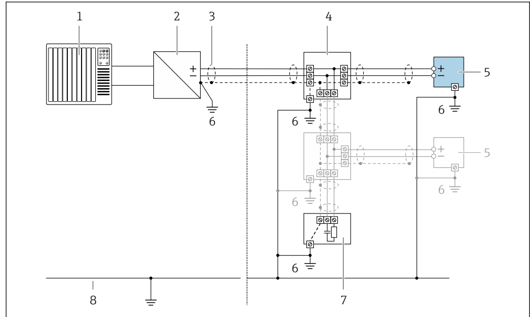
图 14 PROFIBUS PA 的连接实例
