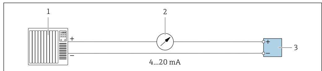
图 15 4...20 mA 有源电流输出的连接实例
