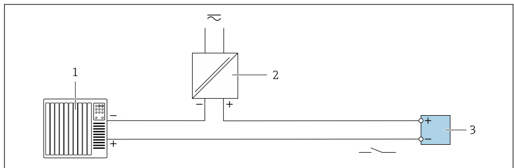
图 19 开关量输出(无源信号)的连接实例
