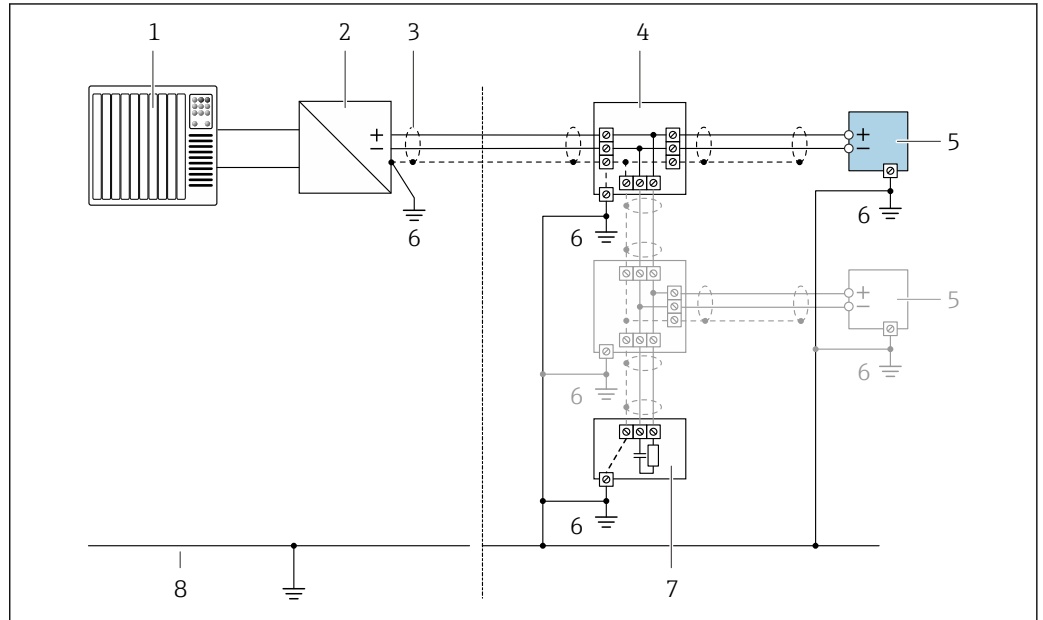
图 15 PROFIBUS PA 的连接实例
