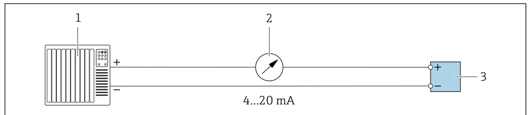
图 16 4...20 mA 有源电流输出的连接实例
