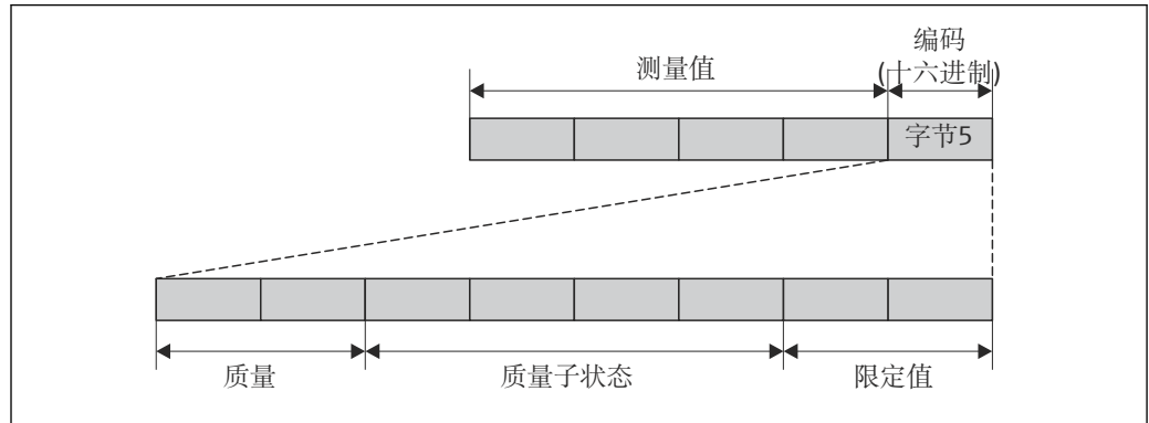
图 33 编码字节的结构
