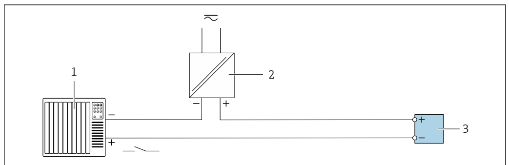
图 22 状态输入的连接实例
