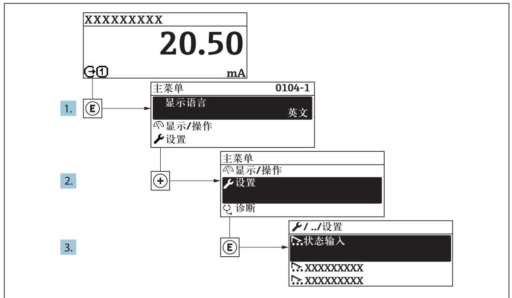
图 29 现场显示单元示例
