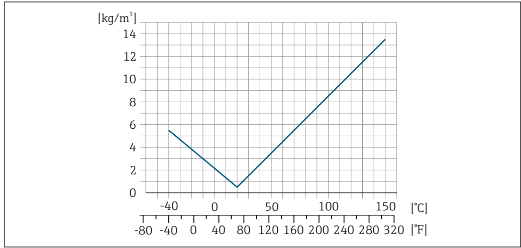
图 24 现场密度标定, 例如: 在+20 °C (+68 °F)时
