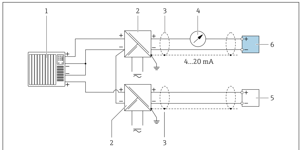
图 11 带公用负载的 HART 无源输入的连接实例
