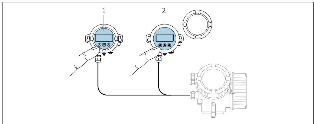
图 27 FHX50 的操作选项
