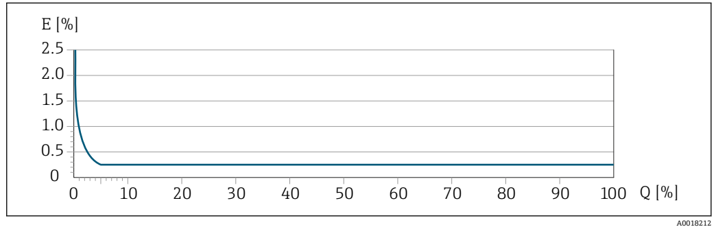
图 25 最大测量误差(% o.r.) (例如: DN 25)
