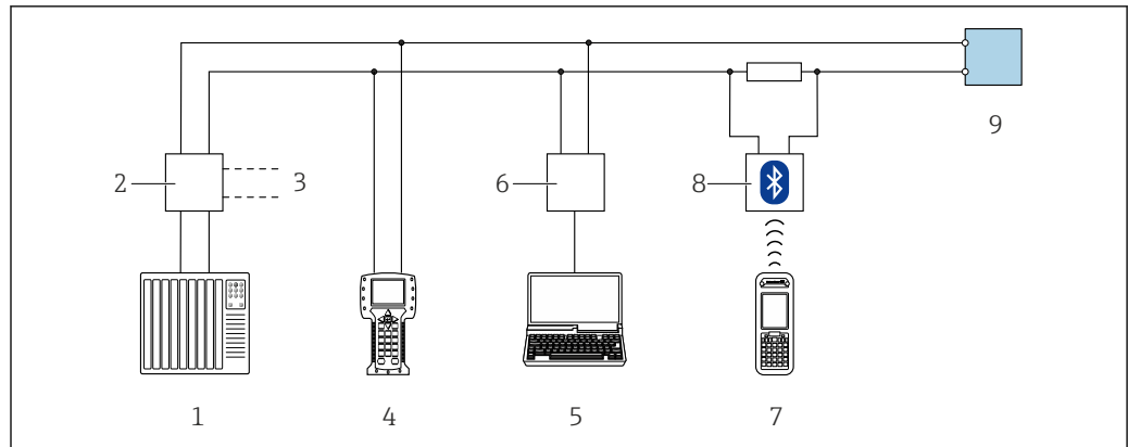
图 14 通过 HART 通信进行远程操作（无源信号）
