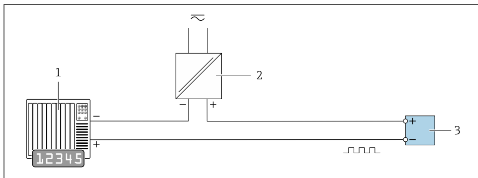
7 Esempio di connessione per uscita impulsi/frequenza (passiva)
