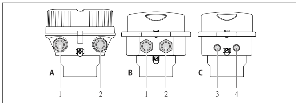
3 Versioni della custodia e versioni della connessione
