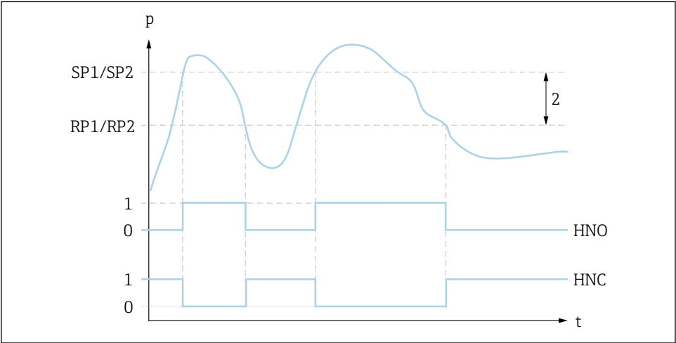
图 1 SP1/SP2: 动作点 1/2; RP1/RP2: 恢复点 1/2
