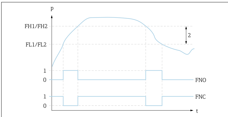
图 2 FH1/FH2: 压力窗口的上限值; FL1/FL2: 压力窗口的下限值
