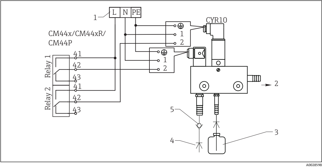
图 36 Chemoclean CYR10 清洗单元接线图
