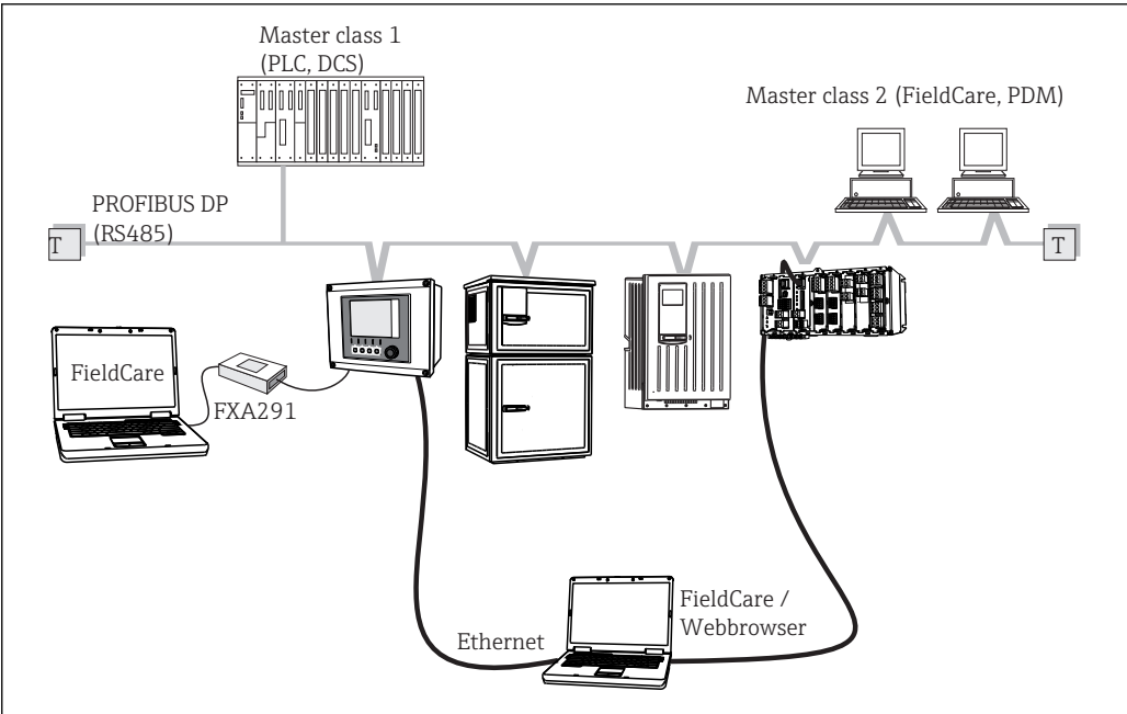
图 12 PROFIBUS DP
