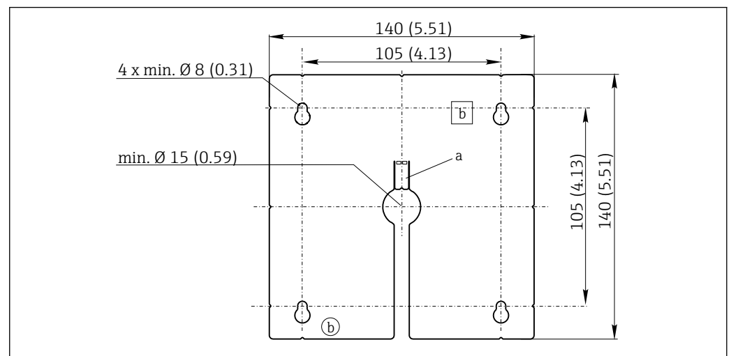
图 9 外接显示单元安装板的外形尺寸示意图, 单位: mm (inch)
