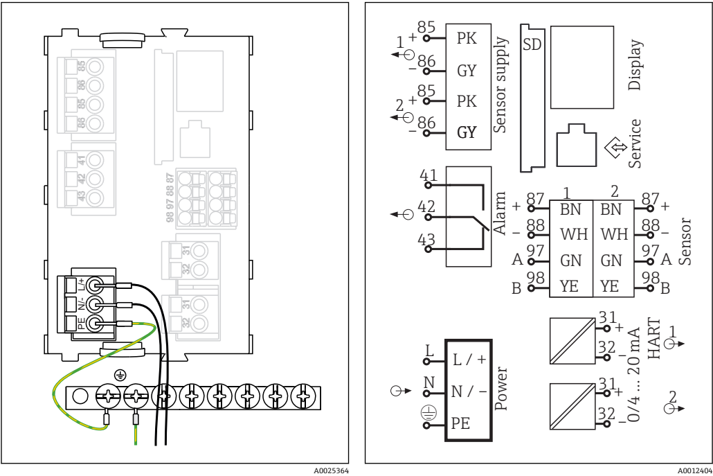
图 15 在 BASE-H 或 BASE-L 模块的接入供电电压 图 16 BASE-H 或-L 模块的完整接线示意图
