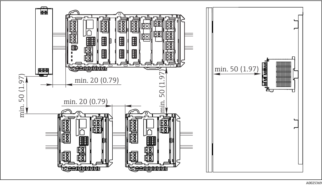
图 7 最小安装间距；单位：mm (inch)
