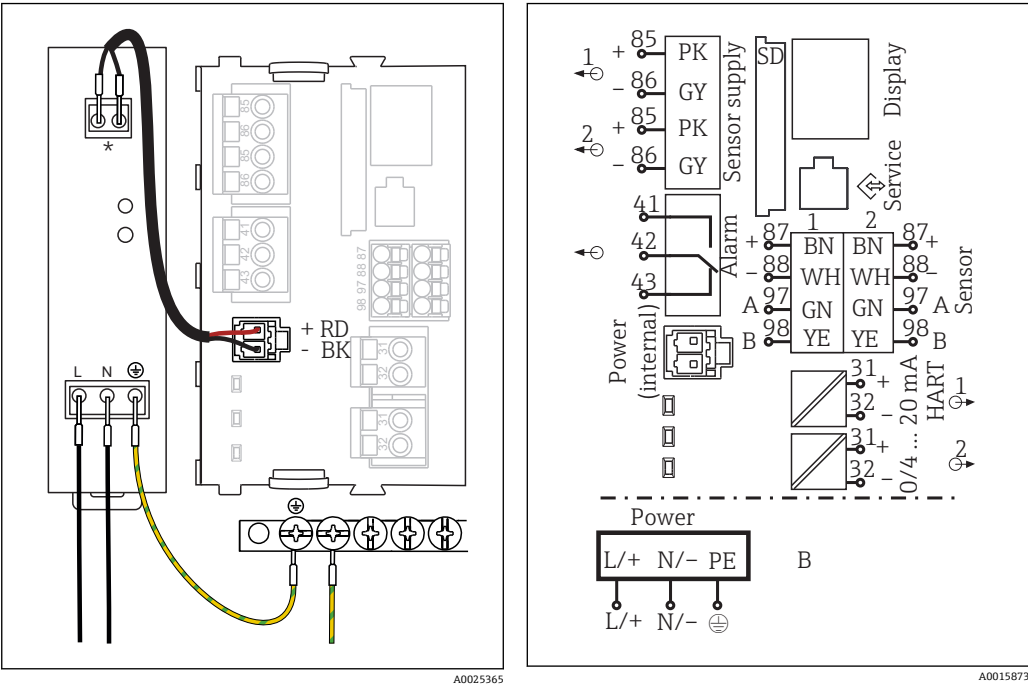
图 17 在 BASE-E 模块上连接电源
