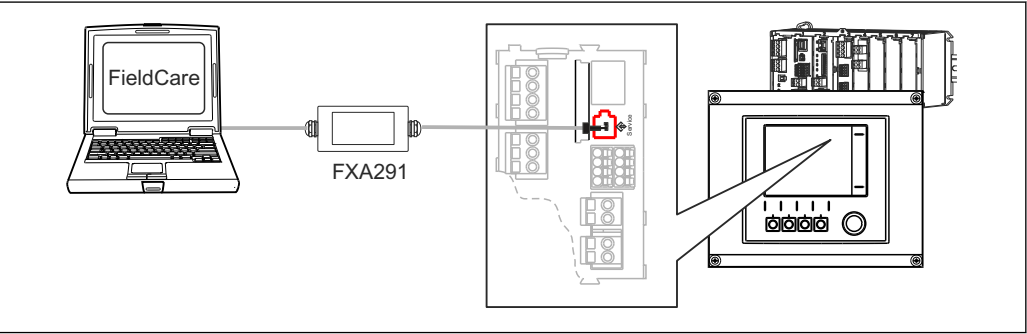
图 48 连接示意图
