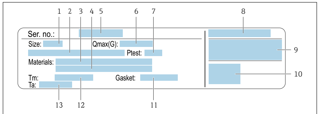
5 Пример заводской таблички датчика
