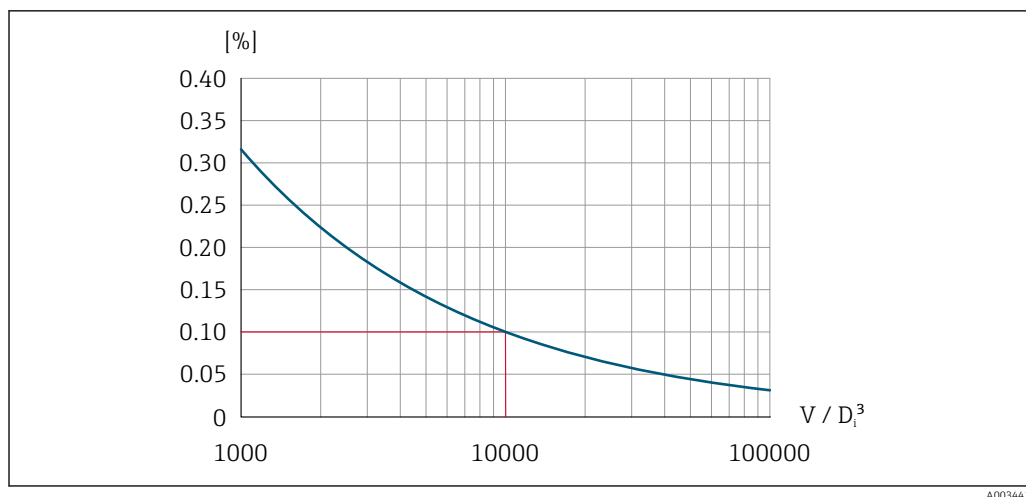
31 Повторяемость = 0,1% ИЗМ при измеренном объемном расходе [м³] V = 1000 \cdot D_i^3
