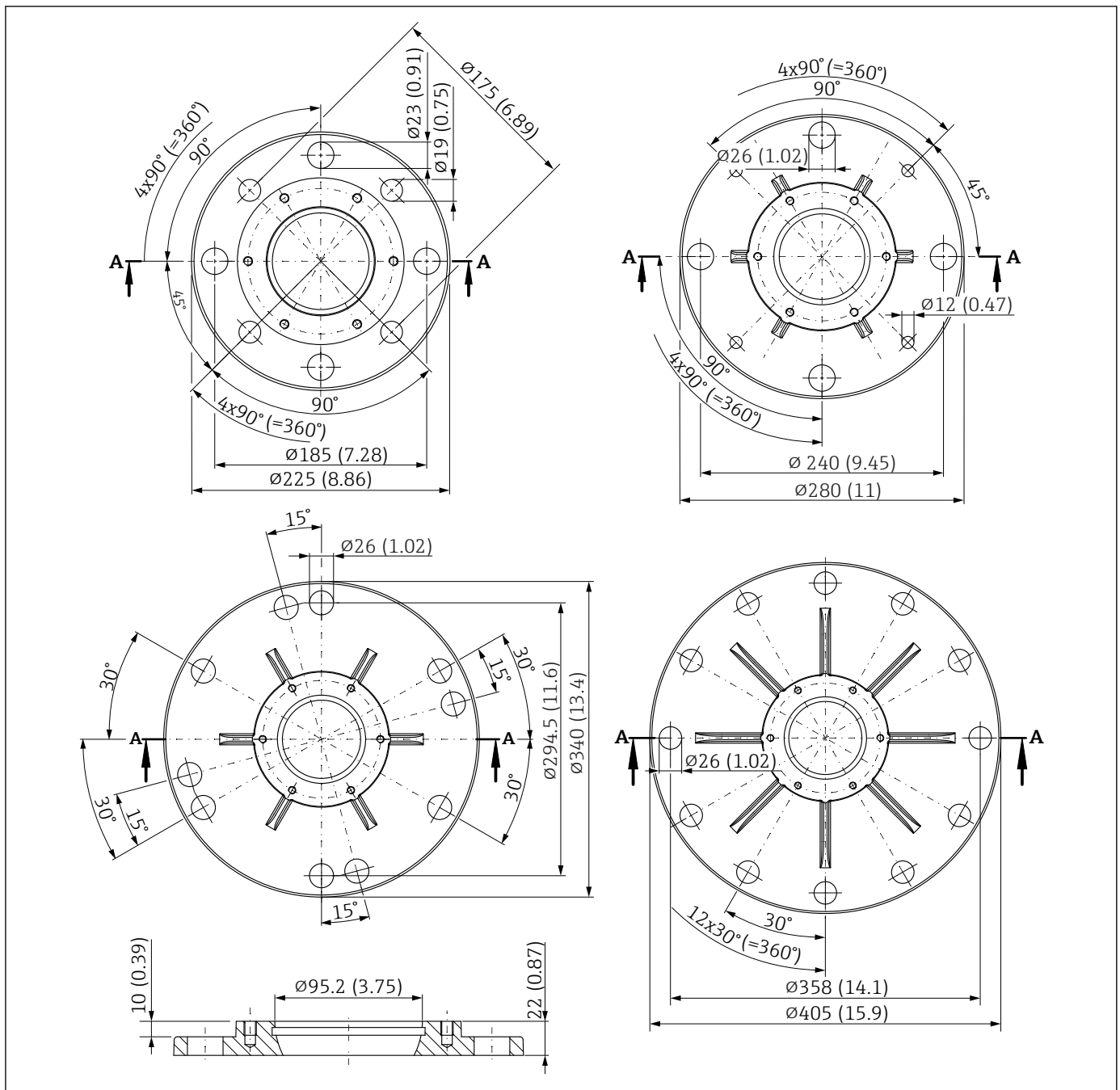
29 FMR67 法兰，带天线角度调节装置；单位：mm (in)
