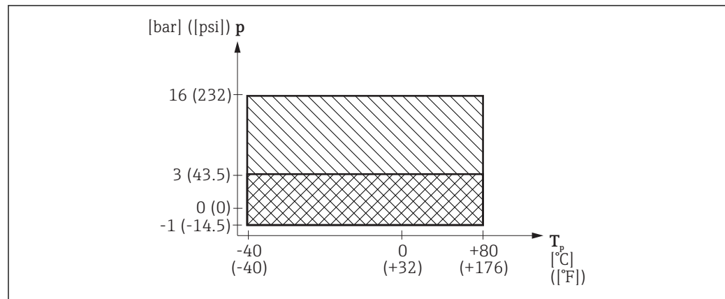
图 14 FMR67: 允许过程温度和过程压力范围，带 PTFE 全填充水滴天线，DN50
