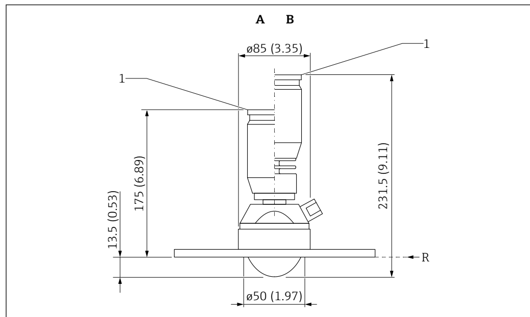
图 26 外形尺寸示意图; 单位: mm (in)
