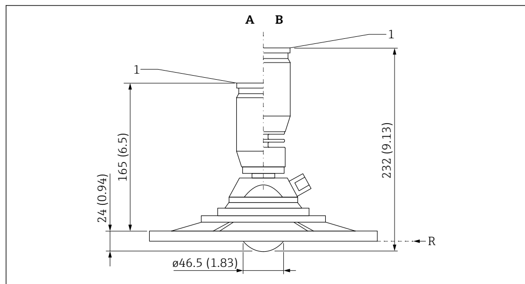
28 外形尺寸示意图; 单位: mm (in)
