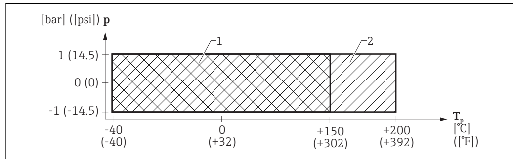
图 17 FMR67: 允许过程温度和过程压力范围, 带 PTFE 全填充齐平安装天线, DN80 和可调节 UNI 法兰, 铝
