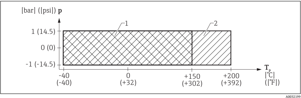
图 16 FMR67：允许过程温度和过程压力范围，带 PTFE 全填充齐平安装天线，DN80 和 UNI 法兰，316L 1 订购选项 90 “密封圈”，选型代号 A5：FKM Viton GLT 2 订购选项 90 “密封圈”，选型代号 A6：FKM Viton GLT
