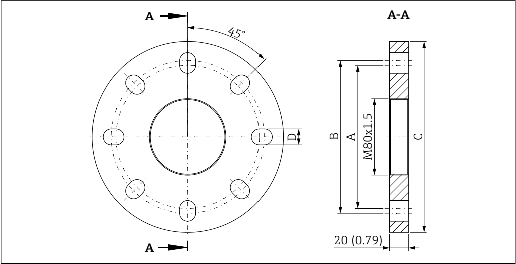
24 外形尺寸示意图；单位：mm (in)
