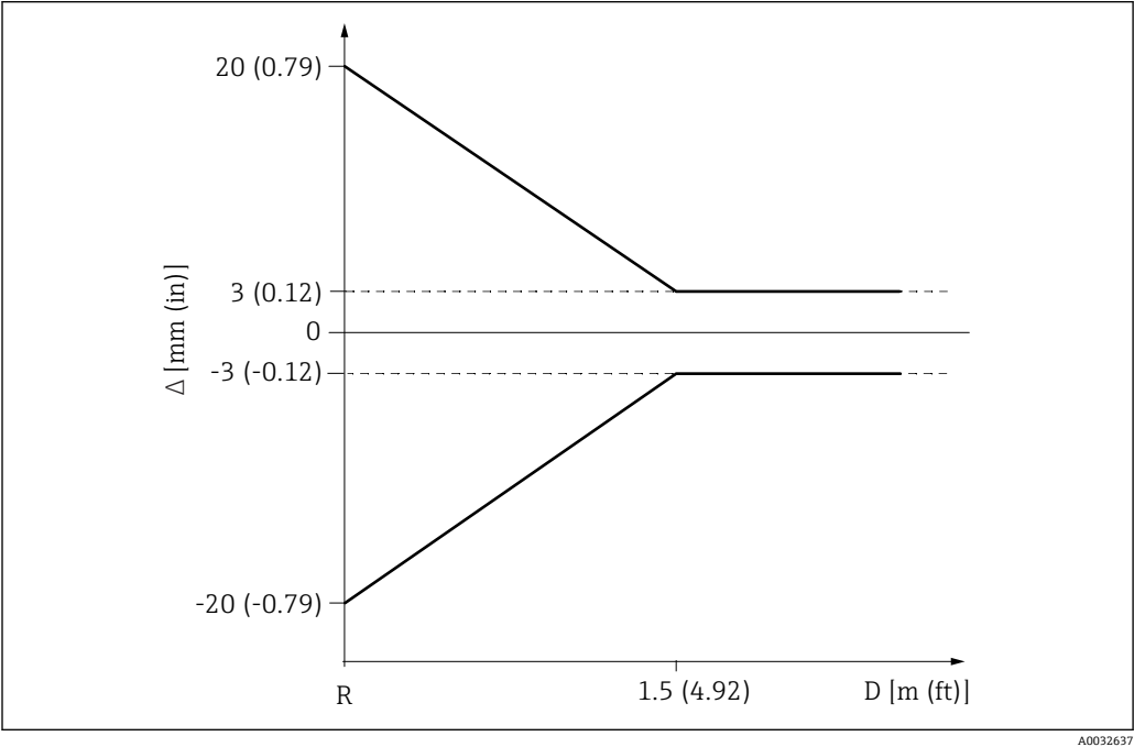
图 11 近距离测量时的最大测量误差
