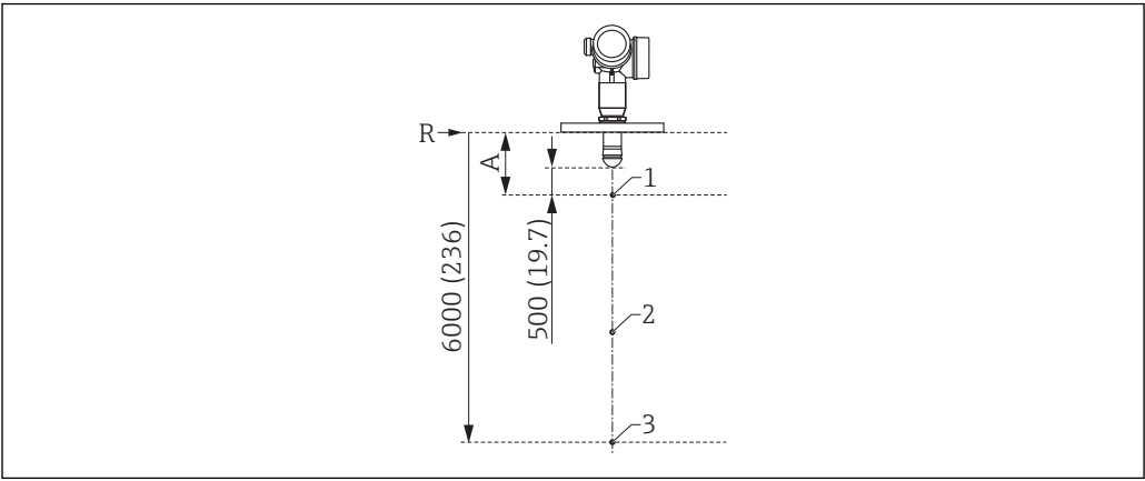
图 37 三点线性标定中的三个标定点的图示说明；单位：mm (in)
