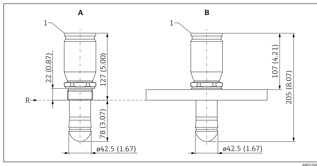
图 21 外形尺寸示意图; 单位: mm (in)
