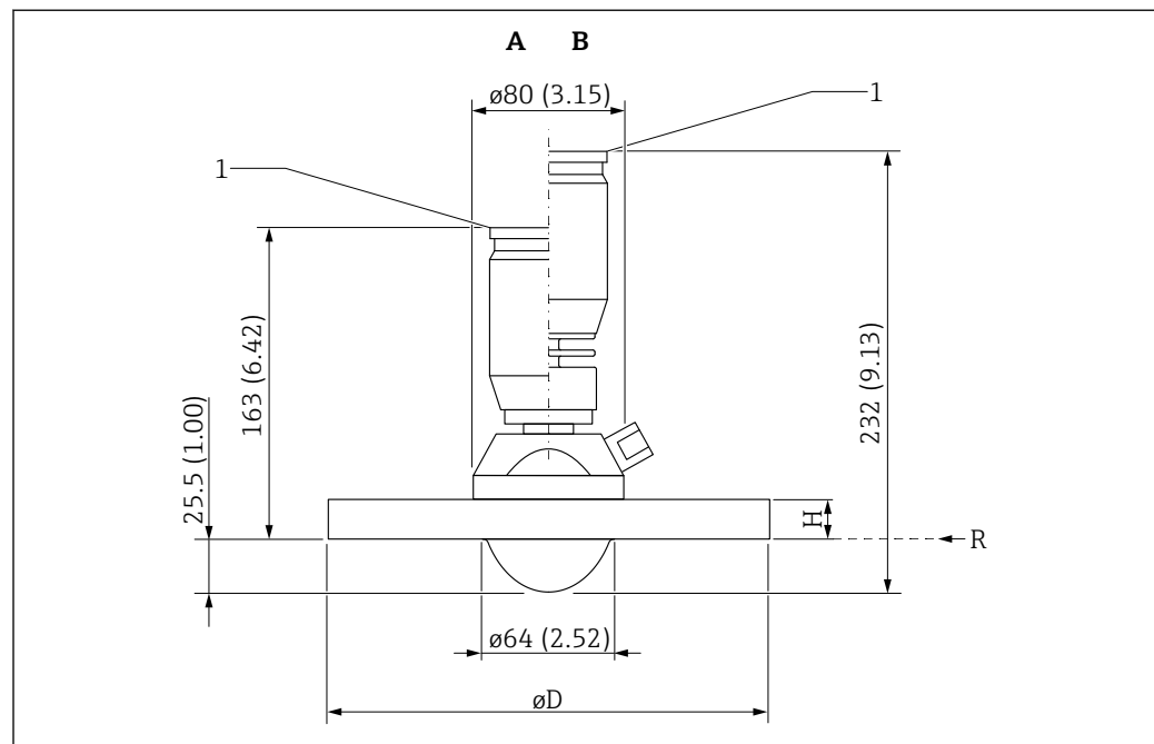
图 25 外形尺寸示意图; 单位: mm (in)
