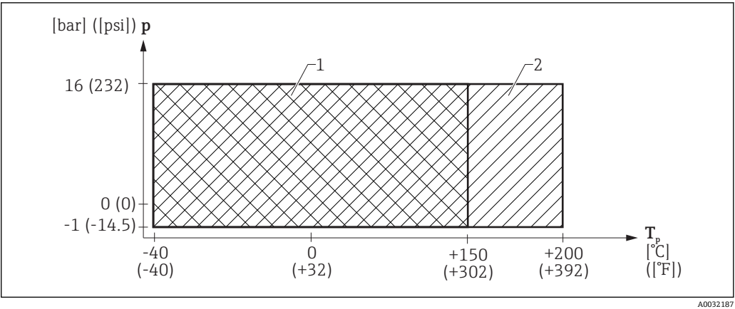
图 15 FMR67：允许过程温度和过程压力范围，带 PTFE 全填充齐平安装天线，DN80 和标准法兰，316L 1 订购选项 90 “密封圈”，选型代号 A5：FKM Viton GLT 2 订购选项 90 “密封圈”，选型代号 A6：FKM Viton GLT
