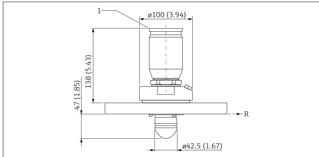
图 23 外形尺寸示意图; 单位: mm (in)
