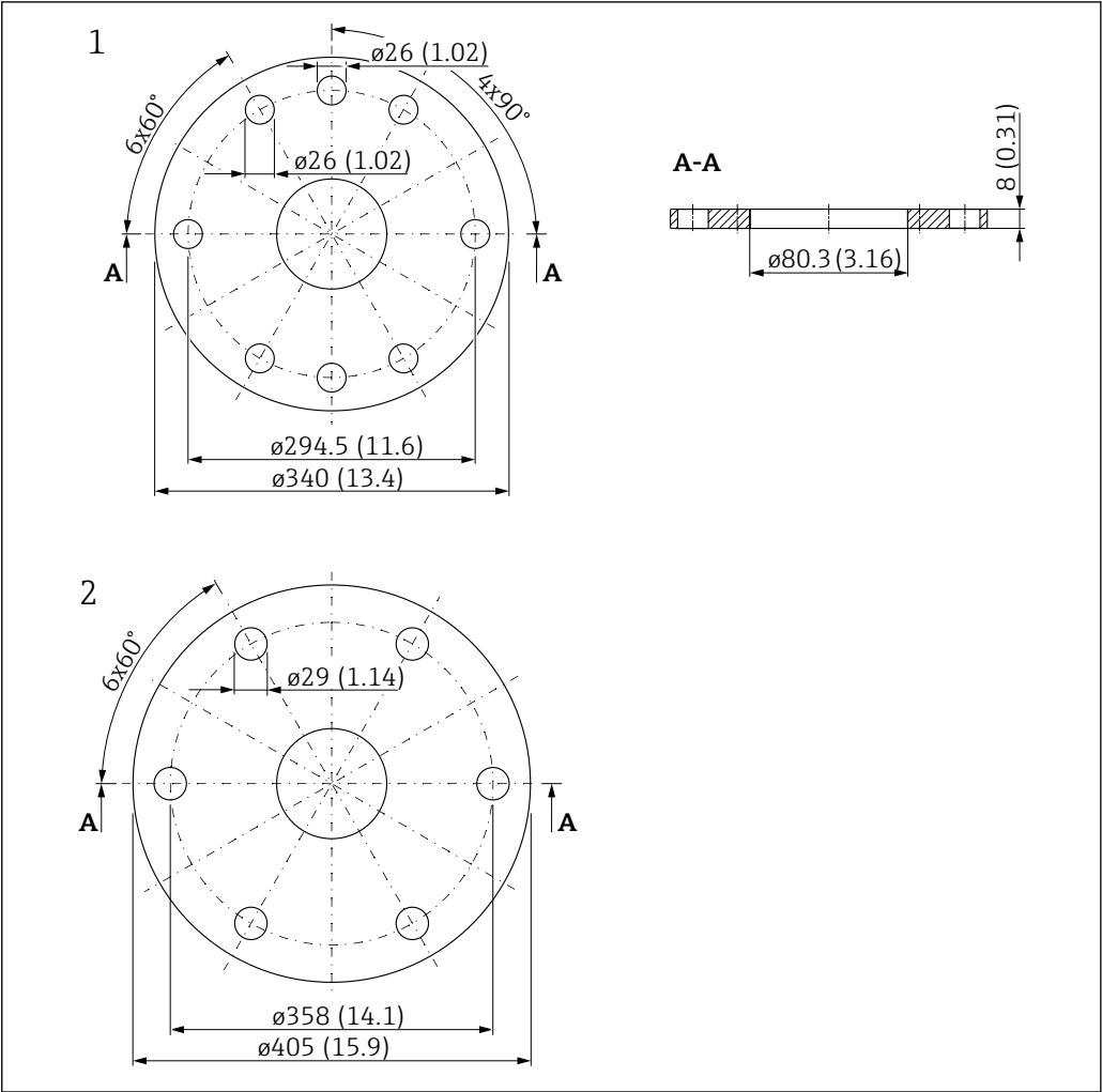
27 外形尺寸示意图；单位：mm (in)
