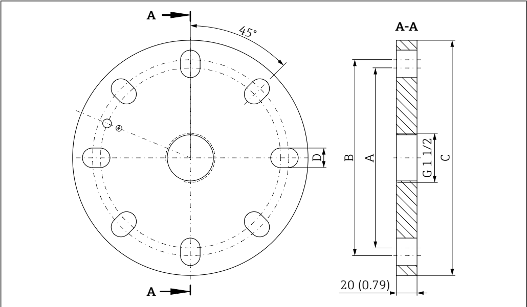
图 22 外形尺寸示意图；单位：mm (in)
