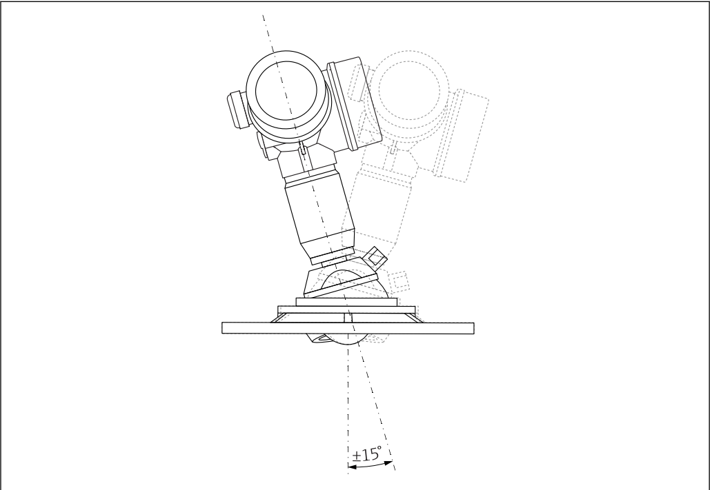
13 带天线角度调节装置的 Micropilot FMR67
