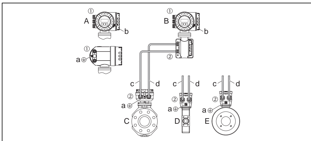
Abb. 12: Construction du système de mesure version compacte / version séparée
