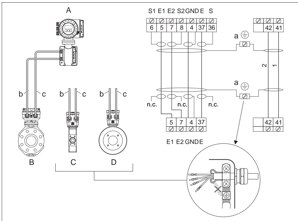
Abb. 14: Connexion câble de raccordement version séparée
