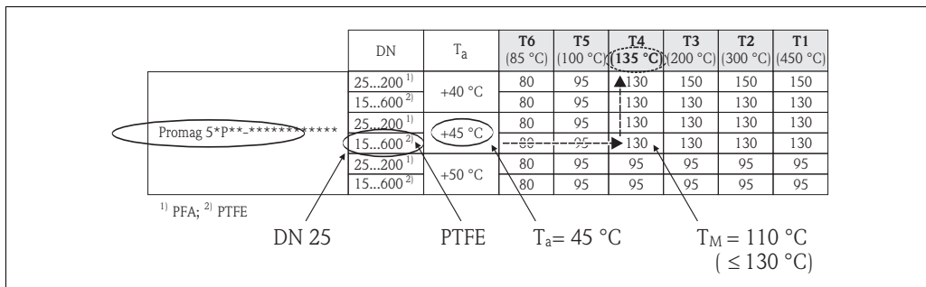
Abb. 1: Vorgehensweise bei Ermittlung der max. Oberflächentemperatur
