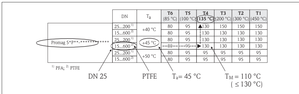
Abb. 11: Procédure pour la détermination de la température maximale de surface
