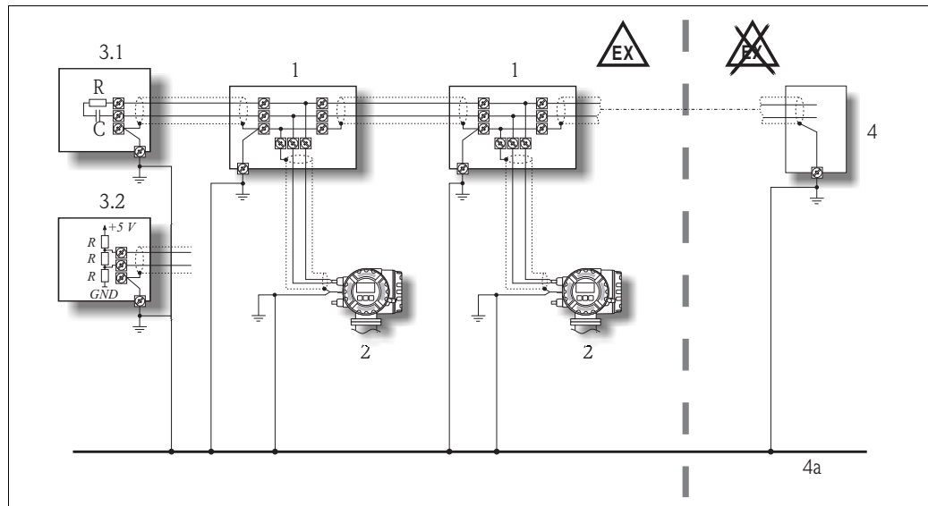
Abb. 13: Exemple de raccordement de câbles d'équipotentialité
