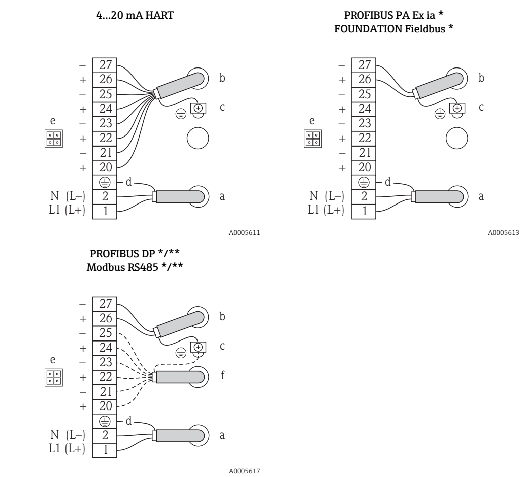
Abb. 15: Raccordements électriques
