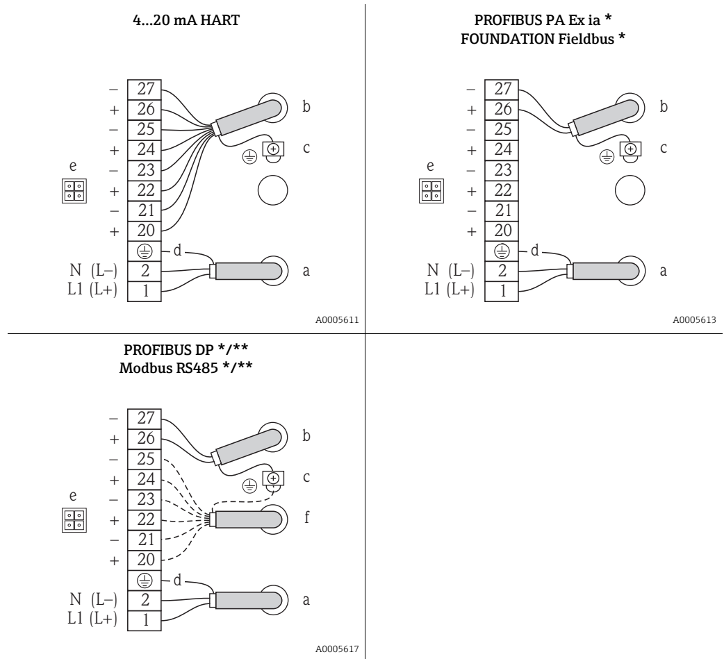
Abb. 5: Elektrische Anschlüsse
