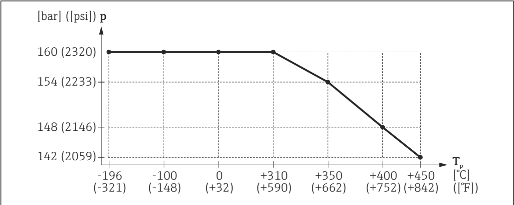
24 FMR51: 高温型仪表的允许过程温度和过程压力范围（订购选项 090 “密封圈”，选型代号 D2）
