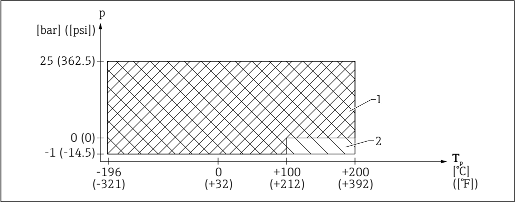
25 FMR52: 允许过程温度和过程压力范围
