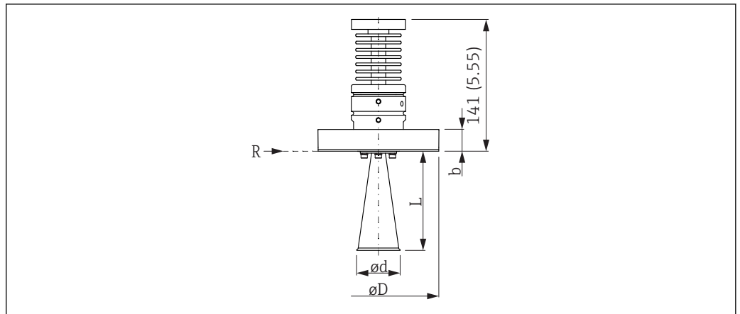
图 32 FMR51 ( T < 450\text{ °C} (842 °F)) 的外形尺寸示意图；单位：mm (in)
