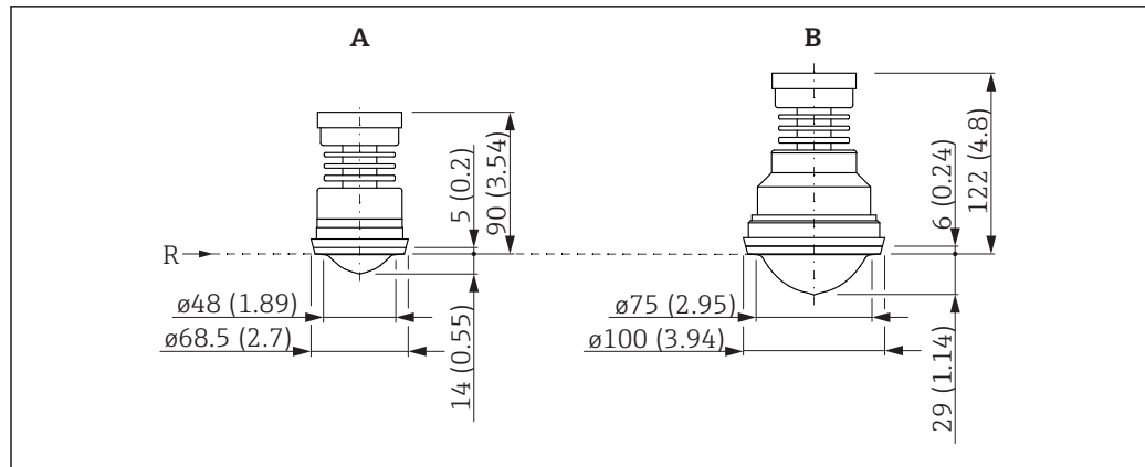
图 33 带 DIN11851 牛奶管道接头的 FMR52 的外形尺寸示意图；单位：mm (in)
