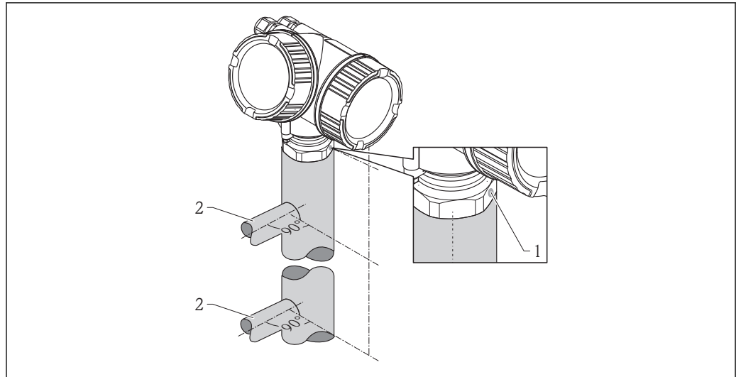
图 22 在旁通管中安装
