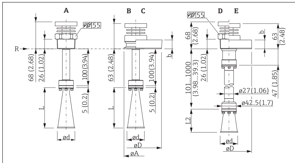
图 30 FMR51 ( T < 150^\circ\text{C} ( 302^\circ\text{F} ), 带天线延伸管) 的外形尺寸示意图; 单位: mm (in)
