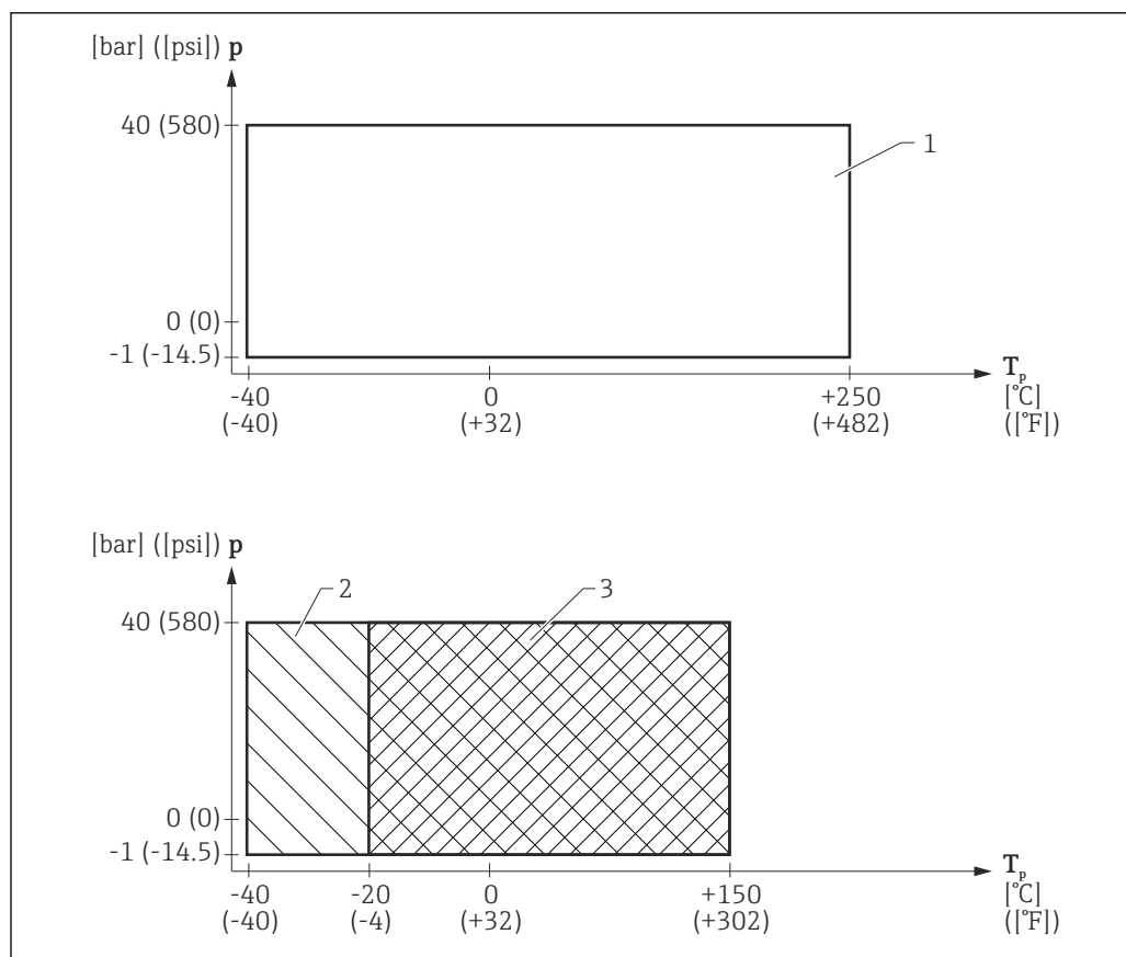
图 23 FMR51: 允许过程温度和过程压力范围
