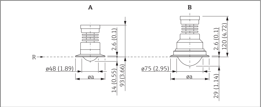
34 带 Tri-Clamp ISO2852 卡箍的 FMR52 的外形尺寸示意图；单位：mm (in)
