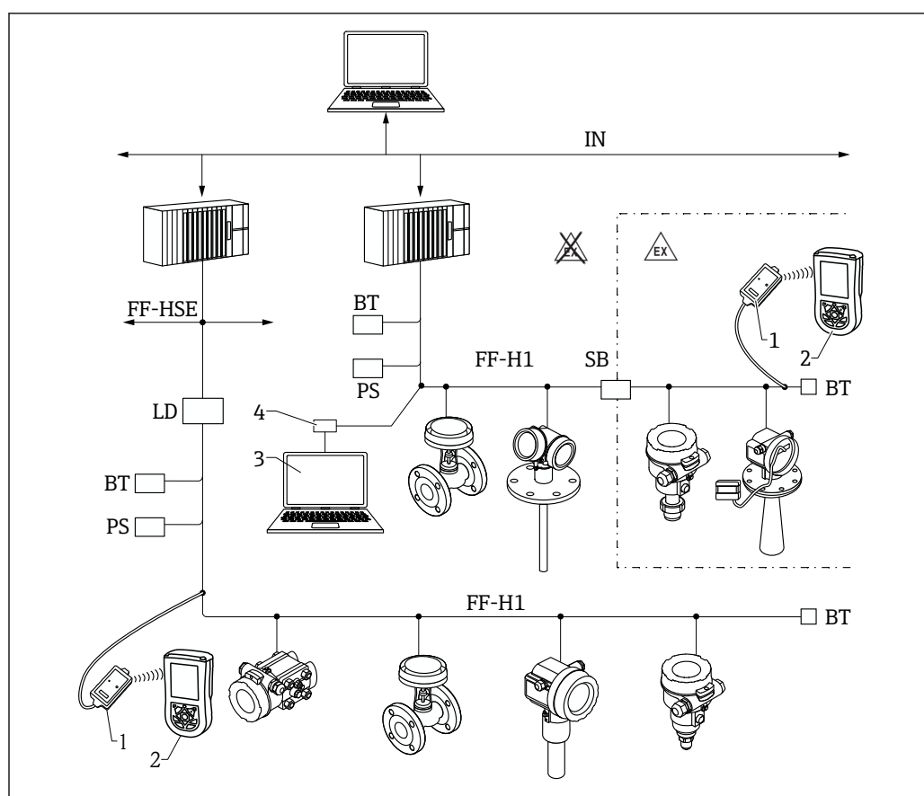
41 FOUNDATION Fieldbus 系统架构及其相关部件
