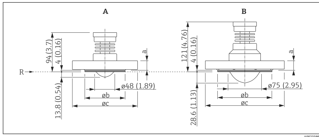
图 35 带法兰的 FMR52 的外形尺寸示意图；单位：mm (in)
