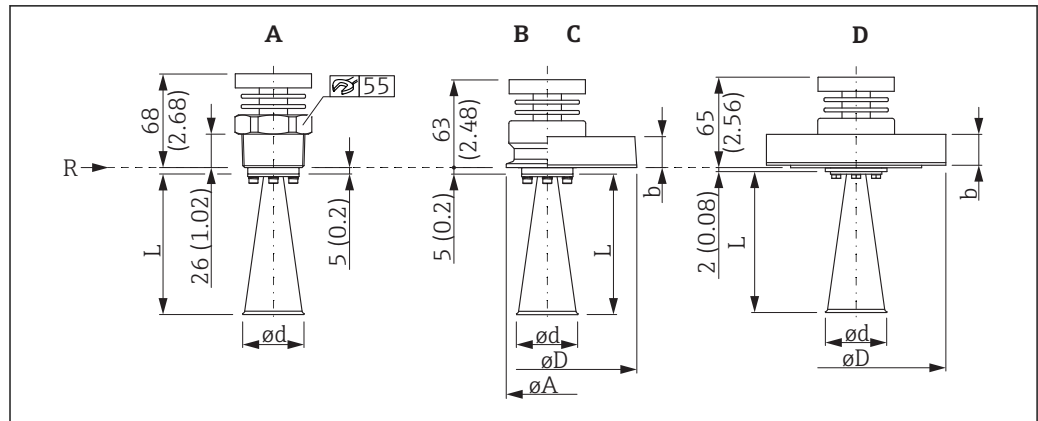
图 29 FMR51 ( T < 150\text{ °C} (302 °F), 无天线延伸管) 的外形尺寸示意图; 单位: mm (in)
