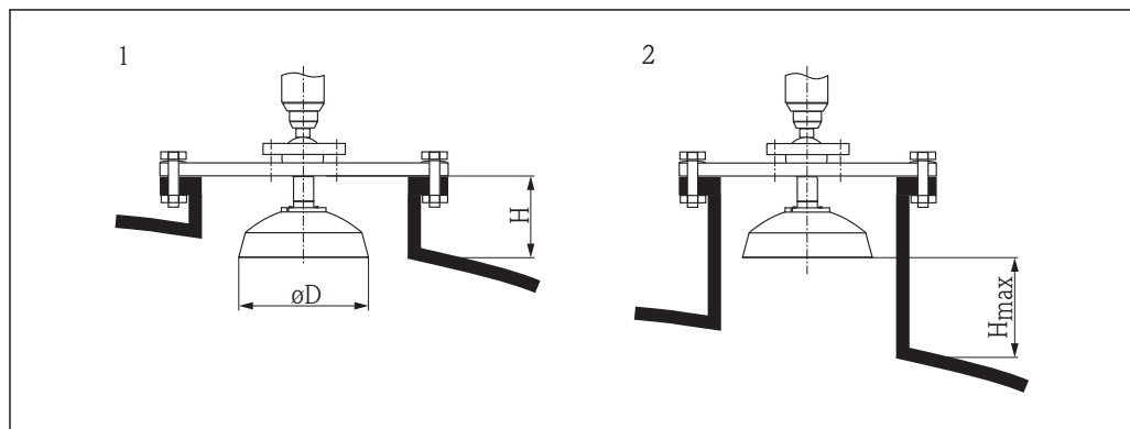
图 21 带抛物面天线的 Micropilot 的安装短管安装示意图
