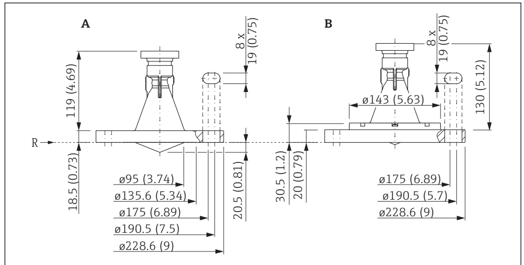
图 32 带 4"/DN100 松套法兰的 FMR56 的外形尺寸示意图；单位：mm (in)
