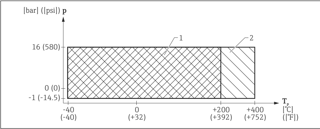
图 25 FMR57: 允许过程温度和过程压力范围
