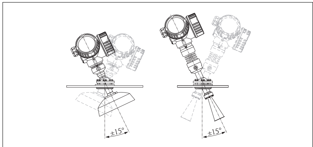
图 22 带天线角度调节装置的 Micropilot FMR57
