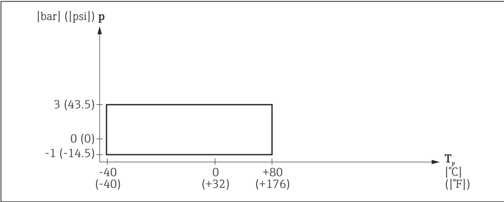
图 24 FMR56: 允许过程温度和过程压力范围
