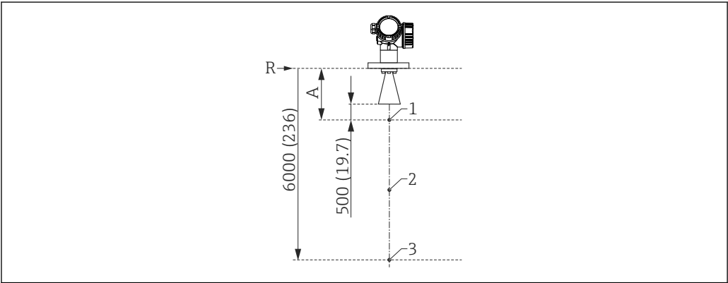
46 三点线性协议中的三个点的示意图; 单位: mm (in) A 参考点 R 至第一个测量点的距离 R 测量参考点 1 第一个测量点 2 第二个测量点 (在第一个和第三个测量点的中间) 3 第三个测量点
