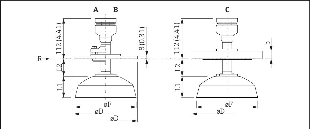
36 带抛物面天线的 FMR57 的外形尺寸示意图；单位：mm (in)
