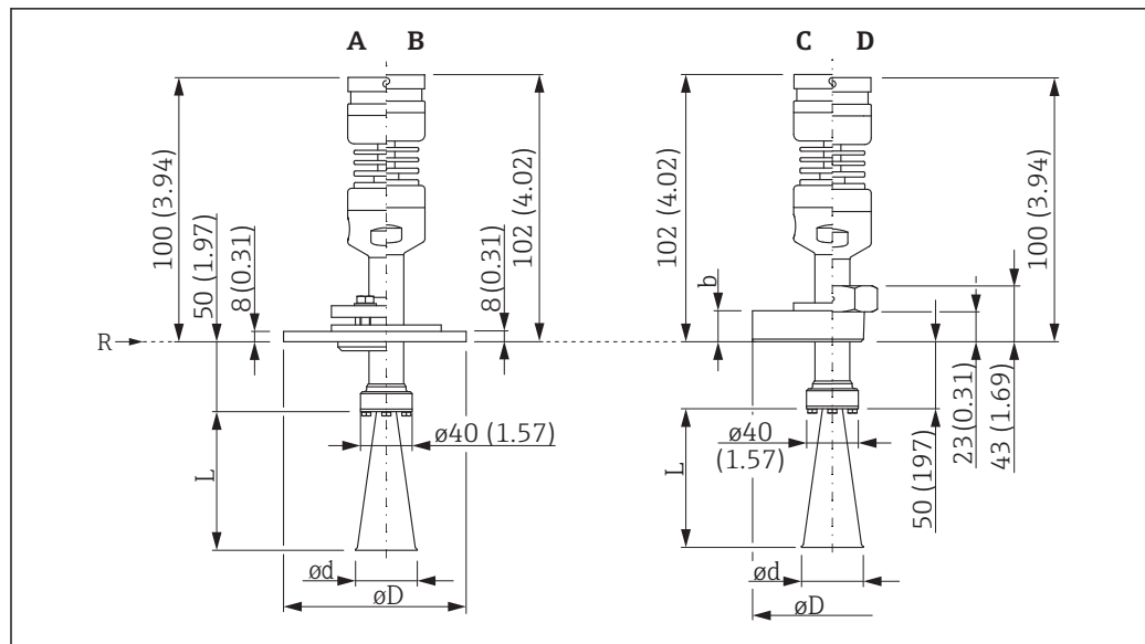
图 35 带喇叭天线的 FMR57 (高温型) 的外形尺寸示意图; 单位: mm(in)
