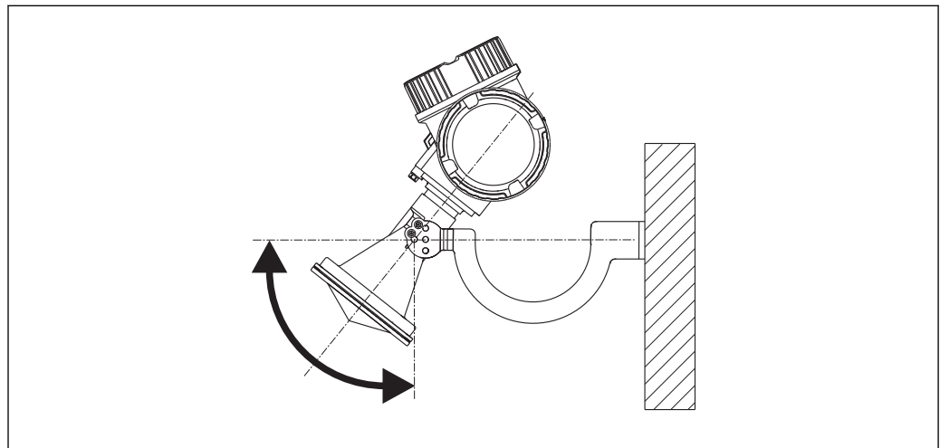
图 19 带安装支架的喇叭天线的安装示意图
