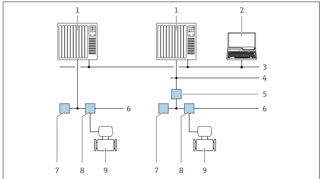
图 17 通过基金会现场总线(FF)网络进行远程操作
