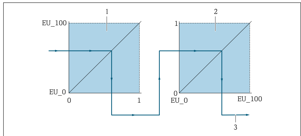
图 22 在模拟量输入块中的比例缩放测量值
