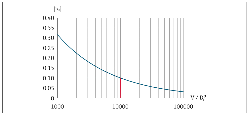
图 27 重复性为 0.1 % o.r., 体积流量测量值[m 3 ]为 V = 1000 · D 1 3
