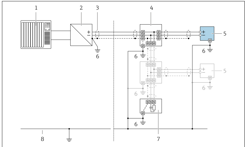
图 11 PROFIBUS PA 的接线实例
