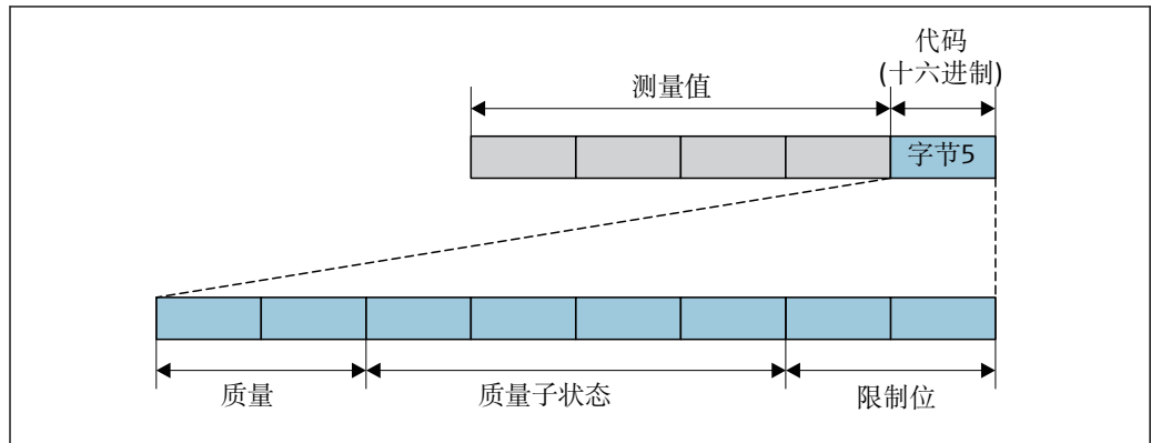
图 23 编码字节的结构
