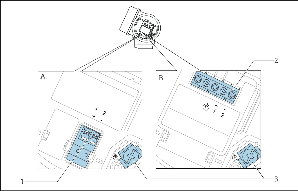
9 接线端子分配: 两线制; 4...20 mA HART
