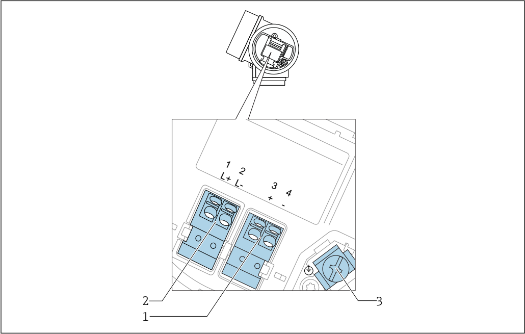
图 15 接线端子分配：四线制；4...20 mA HART (10.4 ... 48 V DC )
