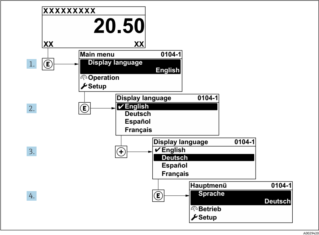
37 现场显示示意图
