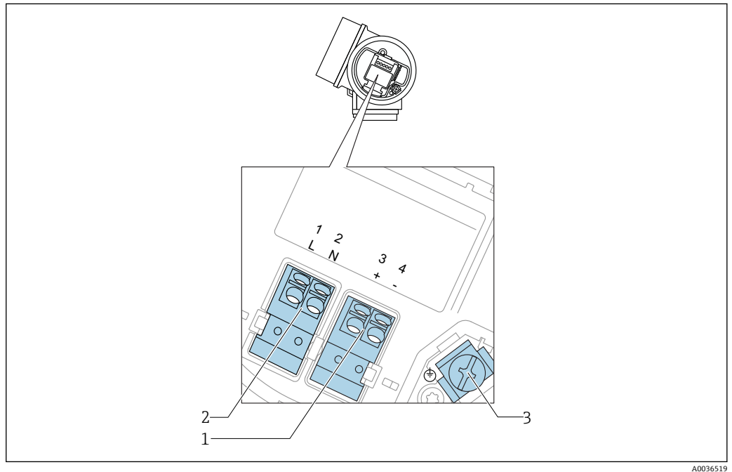
图 17 接线端子分配：四线制；4...20 mA HART (90 ... 253 V AC )
