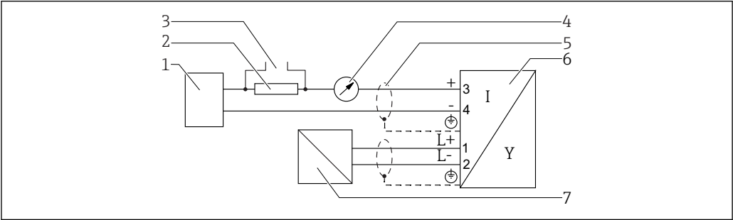
图 16 接线端子分配：四线制；4...20 mA HART (10.4 ... 48 V DC )
