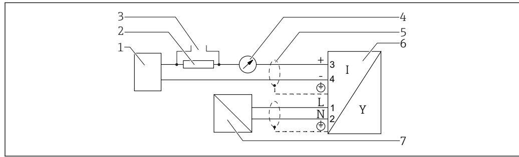
图 18 接线端子分配：四线制；4...20 mA HART (90 ... 253 V AC )
