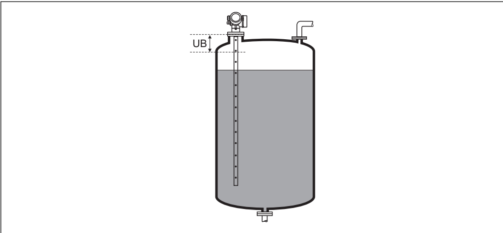
☰ 49 液位测量的盲区距离 (UB)
