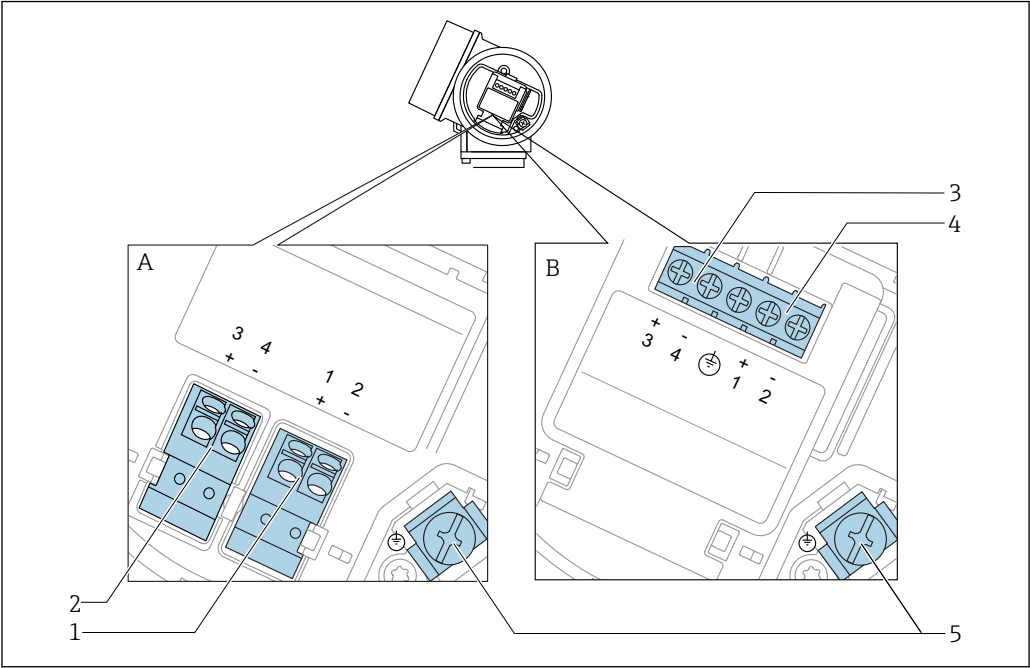
11 接线端子分配：两线制；4...20 mA HART，开关量输出
