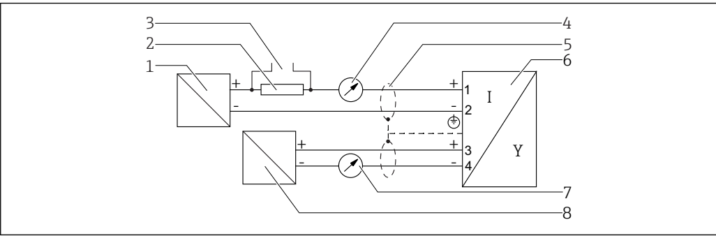
14 接线图：两线制；4...20 mA HART，4...20 mA
