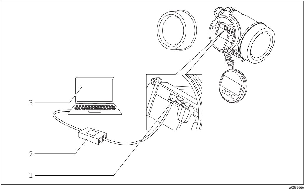
图 27 DeviceCare/FieldCare, 使用服务接口 (CDI)
