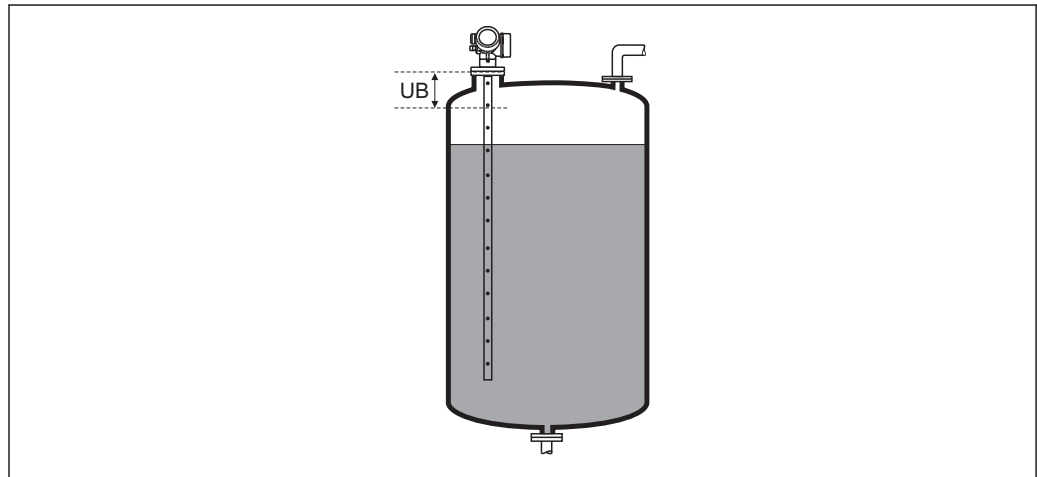
图 52 液位测量的盲区距离 (UB)
