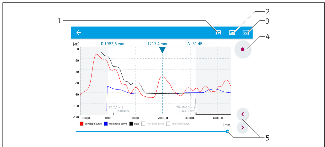
35 在 SmartBlue 中显示包络线；Android 视图
