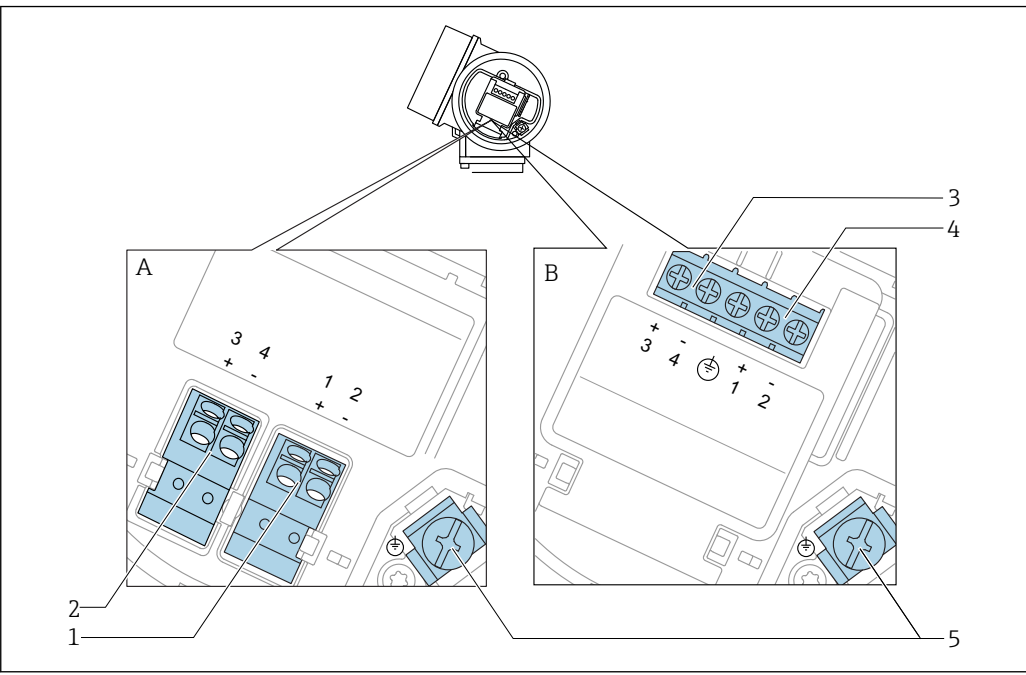
13 接线端子分配：两线制；4...20 mA HART，4...20 mA
