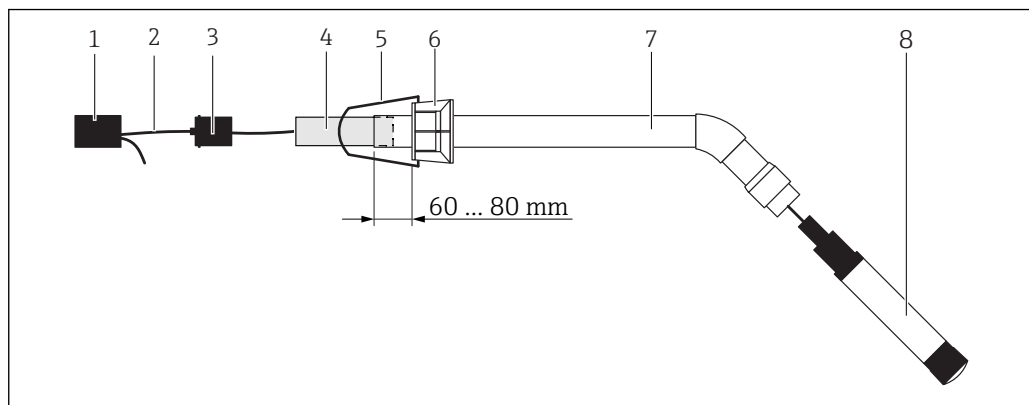
9 Support à immersion CYA112 avec capteur monté
