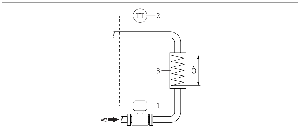
3 Telített gőz vagy víz hőmérséklet-különbségeinek méréseire vonatkozó elrendezés
