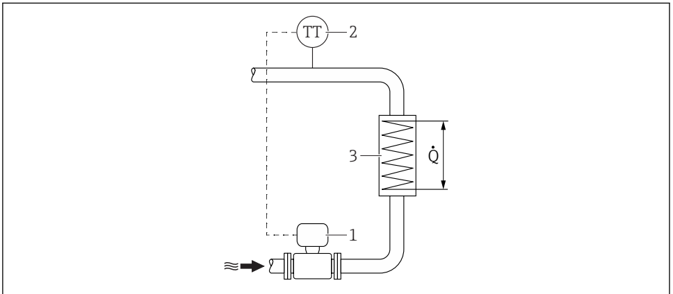
3 Disposizione per misure della differenza di energia del vapore saturo e dell'acqua
