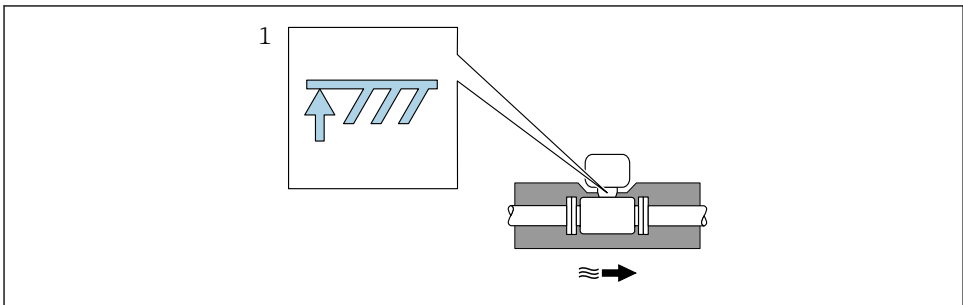
1 Maximale isolatiehoogte
