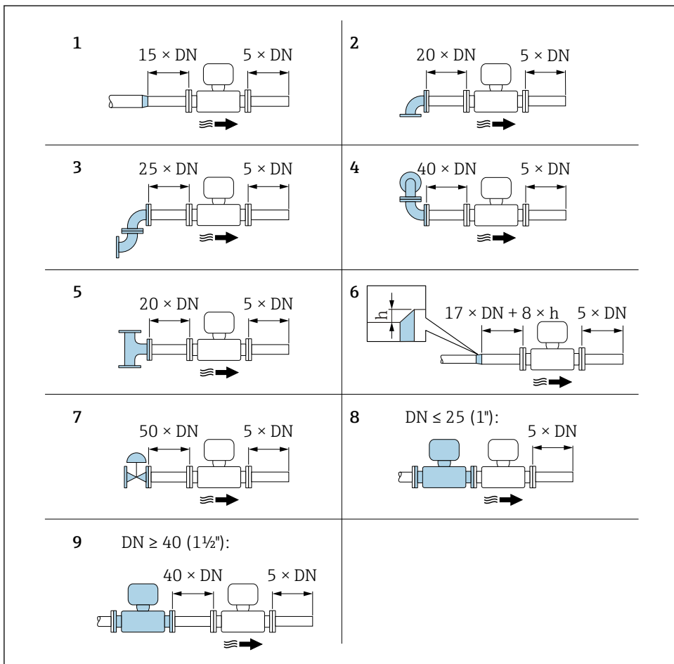
2 Minimalne wymagane długości odcinków dolotowych i wylotowych dla różnych elementów armatury
