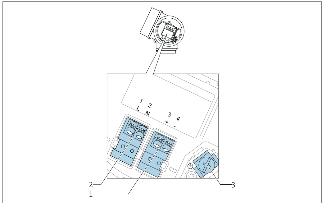
图 11 接线端子分配：四线制；4...20 mA HART (90 ... 253 V AC )
