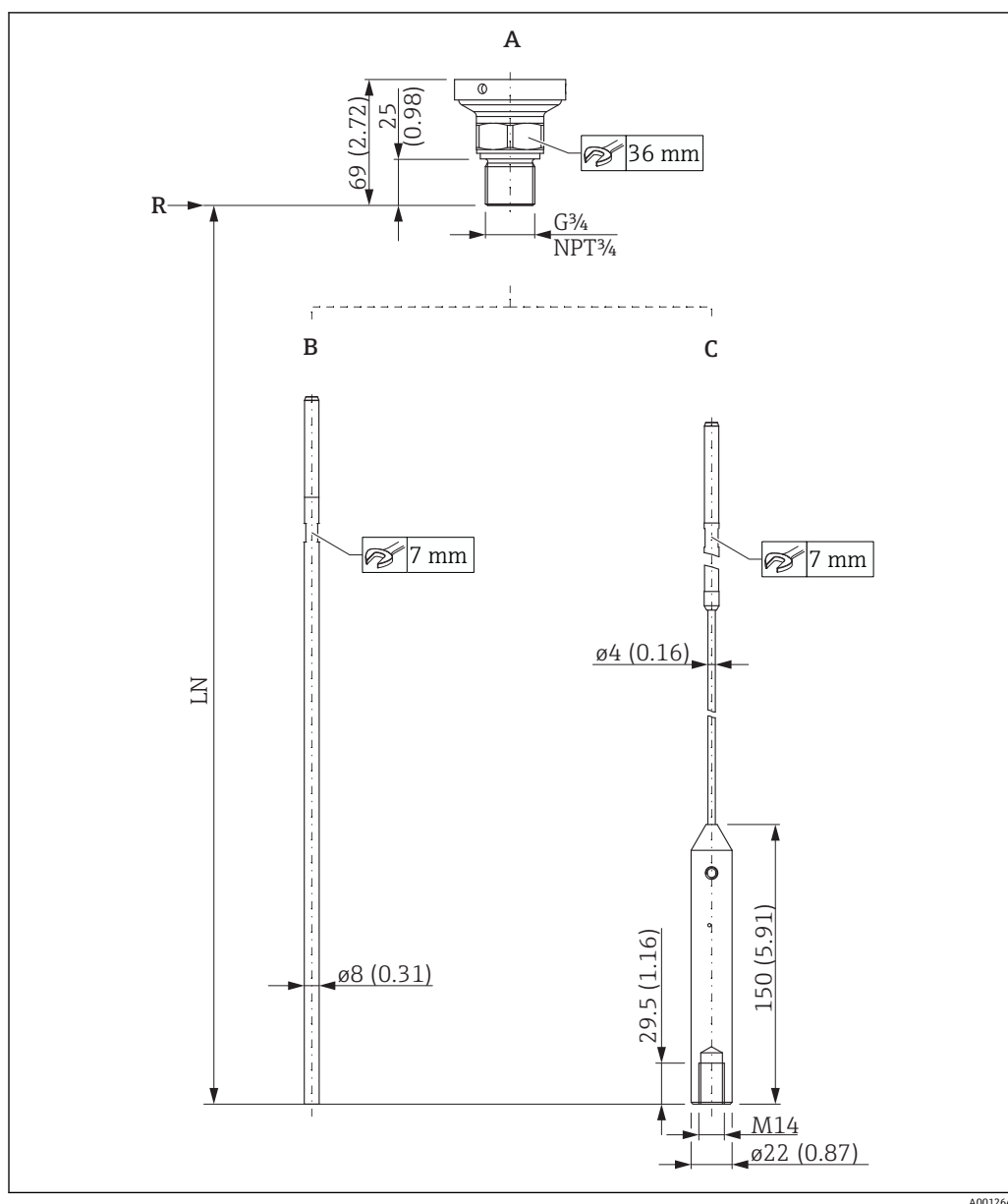
图 27 FMP50: 过程连接/探头。测量单位 mm (in)
