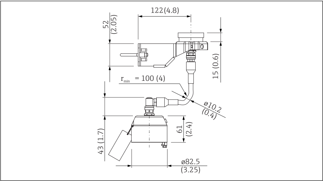
26 分体式探头连接部分；订购的连接电缆长度。测量单位 mm (in)
