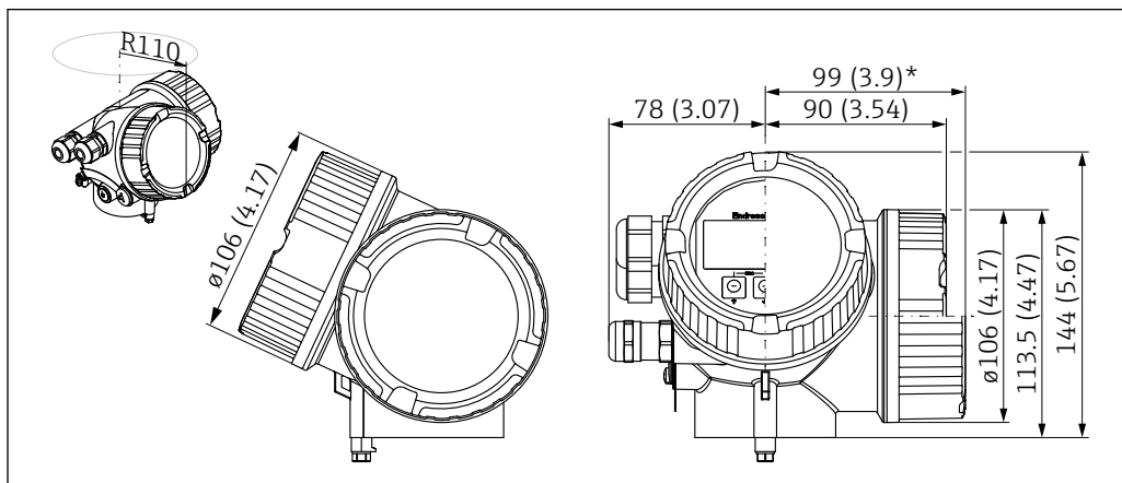
图 23 GT19 外壳 (塑料 PBT) ; 单位: mm (in)
