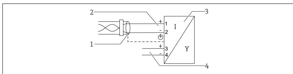
14 接线图: PROFIBUS PA / FOUNDATION Fieldbus
