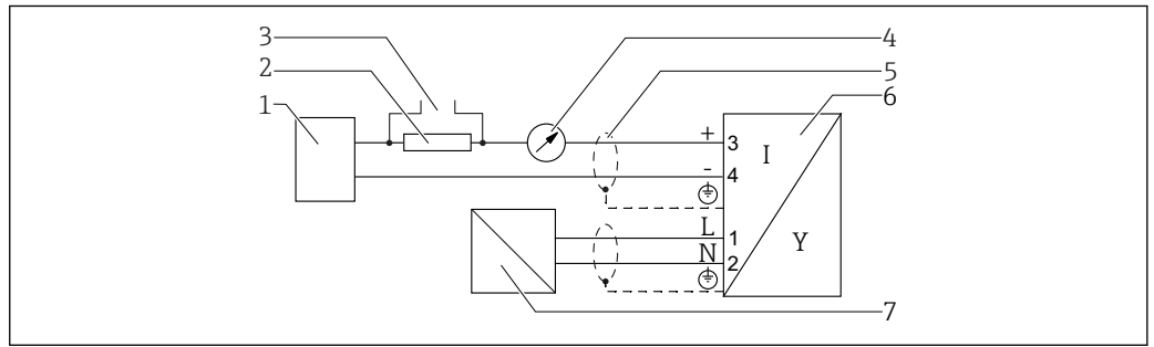
12 接线端子分配: 四线制; 4...20 mA HART (90 ... 253 V AC )
