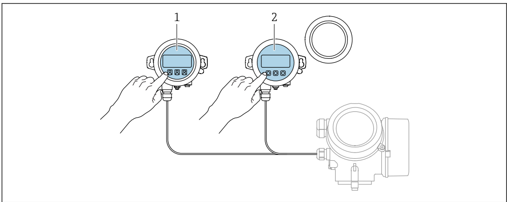
图 28 FHX50 的操作选项 1 显示与操作单元 SD03, 光敏键操作, 可以在玻璃盖板外部操作 2 显示与操作单元 SD02, 按键操作; 必须打开盖板
