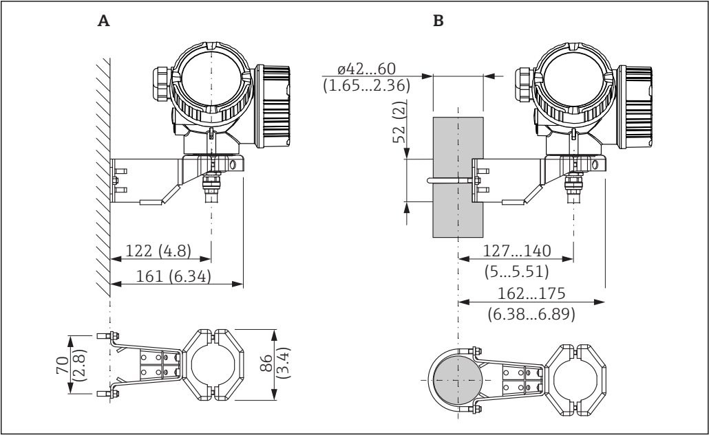
25 电子腔外壳的安装架。测量单位 mm (in)
