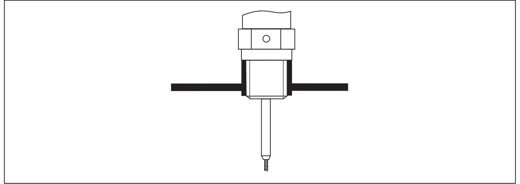
图 21 安装带螺纹连接的仪表；与容器顶齐平安装
