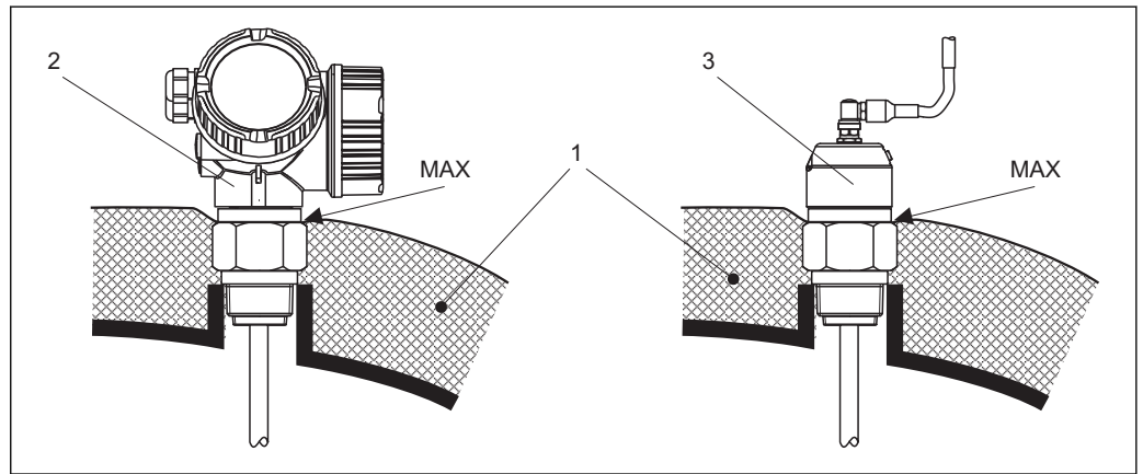
图 22 带螺纹过程连接的 FMP50
