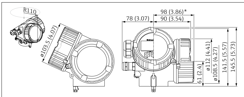
图 24 GT20 外壳 (铝, 带涂层) ; 单位: mm (in)
