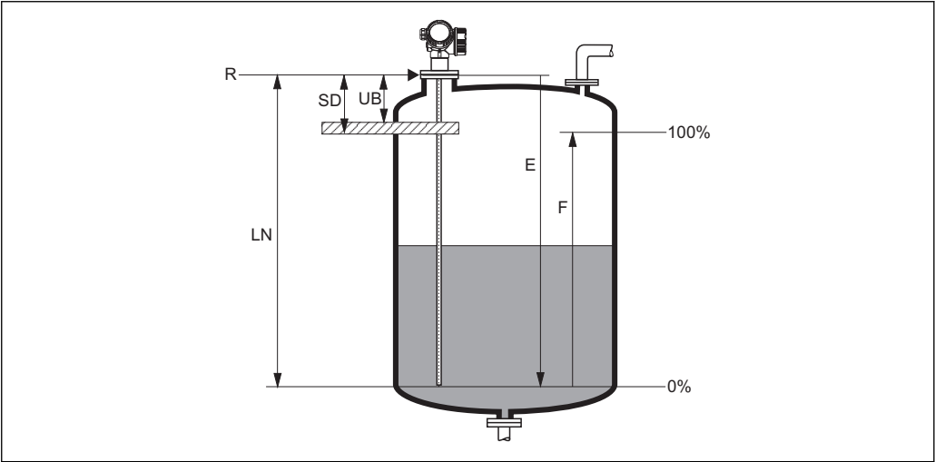
图 2 确定盲区距离和安全距离
