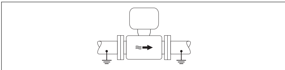
图 1 通过测量管实现电势平衡
