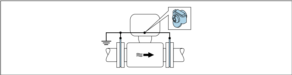
图 3 通过接地端子和接地环实现系统电势平衡
