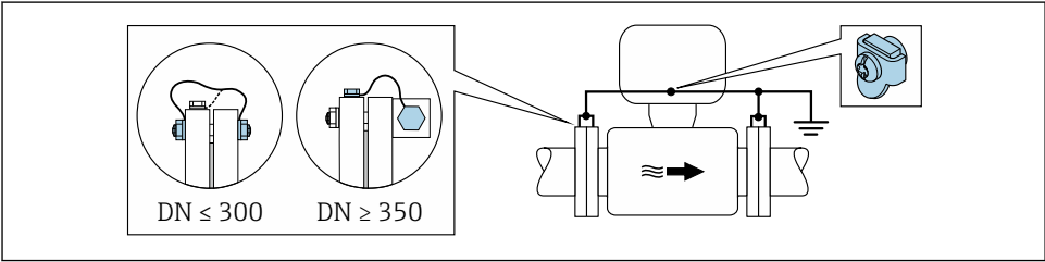
图 2 通过接地端子和管道法兰实现电势平衡
