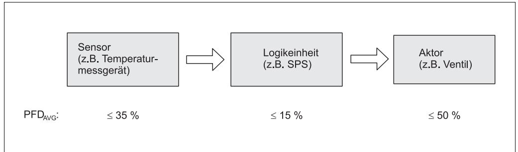
Abb. 1: Übliche Aufteilung der "mittleren Wahrscheinlichkeit gefährdender Ausfälle einer Sicherheitsfunktion im Anforderungsfall" ( PFD_{AVG} ) auf die Teilsysteme
