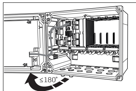
11 Öppna husets kåpa, max. öppningsvinkel 180° (beroende på installationsläge)
