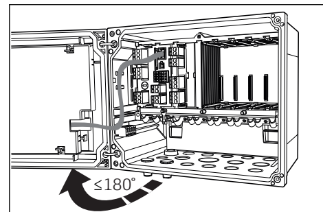
11 Kotelon kannen avaaminen, maks. avauskulma 180^\circ (riippuu asennuspaikasta)
