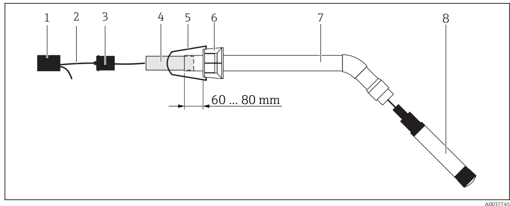
9 Upotusasetelma CYA112, johon on asennettu anturi
