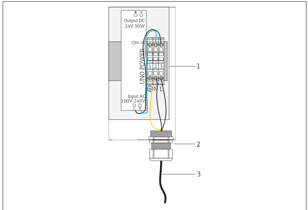
19 Syöttöjännitteen 100...240 V AC kytkeminen
