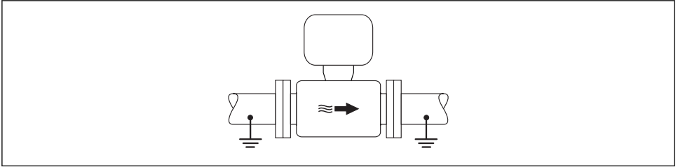
1 Potentialutjämning via mätröret
