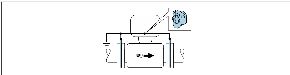
4 Ochranné pospojování přes zemnicí svorku a zemnicí disky
