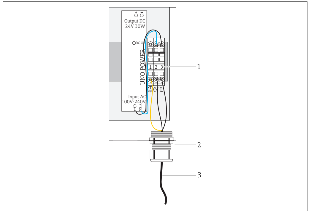
19 Conectarea tensiunii de alimentare 100 până la 240 V CA
